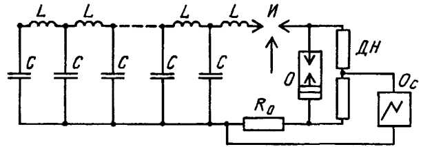
C, L — емкости и индуктивности генератора импульсов тока большой длительности соответственно; И — управляемый искровой промежуток; R_d — шунт для измерения тока; О — испытуемый образец или разрядное сопротивление; ДН — делитель напряжения; Ос — осциллограф
