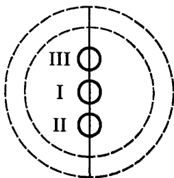
I — рабочее положение нивелира; II — наклонное положение нивелира на угол v_{(+)} ; III — наклонное положение нивелира на угол v_{(-)}
