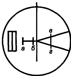
Рисунок 1 — Вид поля зрения окуляра нивелира
