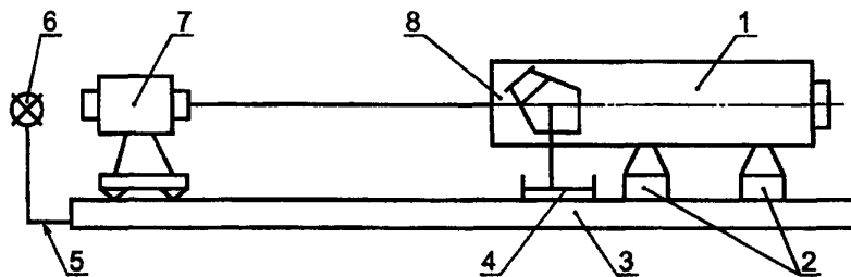
Рисунок А.1 — Поверка нивелира на эталонном компараторе
