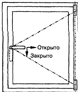
Рисунок А.1 — Устройство по- воротное
