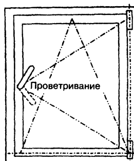
Рисунок А.4 — Устройство по- воротное (откидное, поворотнo- откидное) с функцией регули- руемого проветривания
