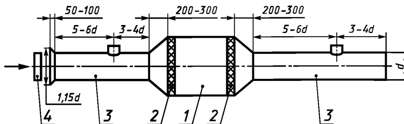
1 — кондиционер; 2 — уплотнение; 3 — измерительная труба; 4 — дозатор пыли (пылепитатель); d — диаметр измерительной трубы
