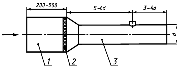
1 — испытуемый прибор; 2 — уплотнение; 3 — измерительная труба; d — диаметр измерительной трубы
