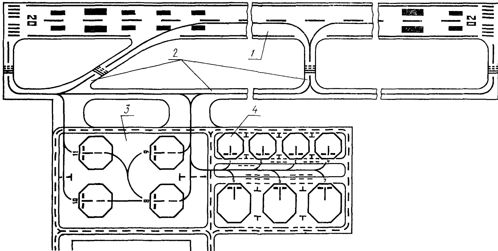
1—искусственная взлетно-посадочная полоса; 2— рулежные дорожки; 3—перрон; 4—места стоянки Черт. 1
