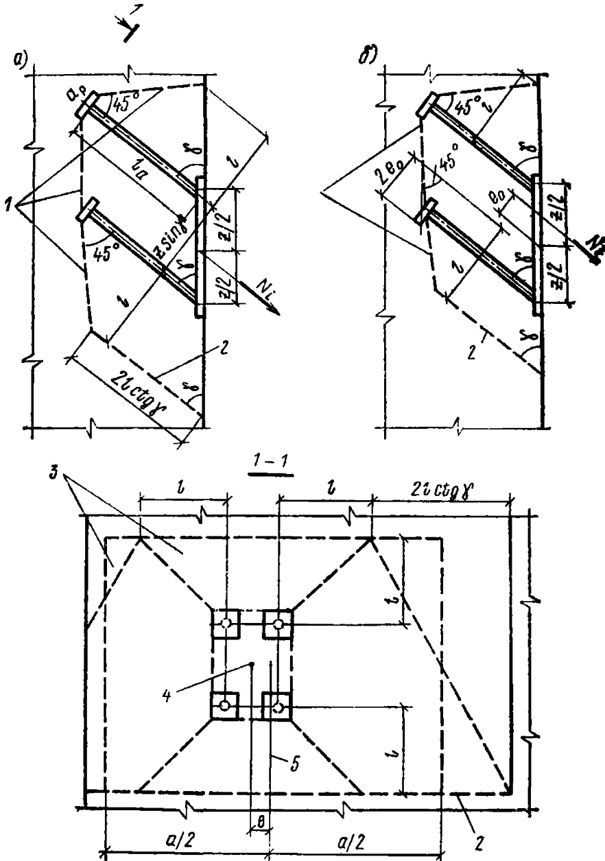
Рис. 12. Схема выкалывания бетона наклонными анкерами при N'_{an} < 0 а — при отсутствии эксцентриситета силы N_i относительно центра тяжести анкеров; б — при наличии такого же эксцентриситета; 1 — поверхность выкалывания; 2 — поверхность среза; 3 — проекция поверхности выкалывания на плоскость, нормальную к анкерам; 4 — точка приложения силы N_i ; 5 — линия центра тяжести площади A_i
