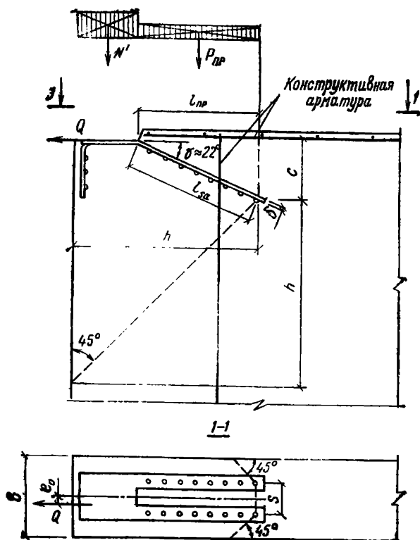
Рис. 19. К расчету штампованной закладной детали при приложении к ней силы Q с эксцентриситетом
