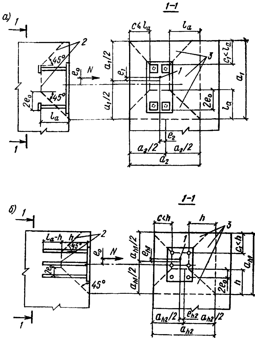
Рис. 9. Схема выкалывания бетона анкерами закладной детали а — с усилениями на концах при N'_{an} < 0 ; б — без усиления на концах при N'_{an} < 0 ; 1 — точка приложения нормальной силы N ; 2 — поверхность выкалывания; 3 — проекция поверхности выкалывания на плоскость, нормальную к анкерам
