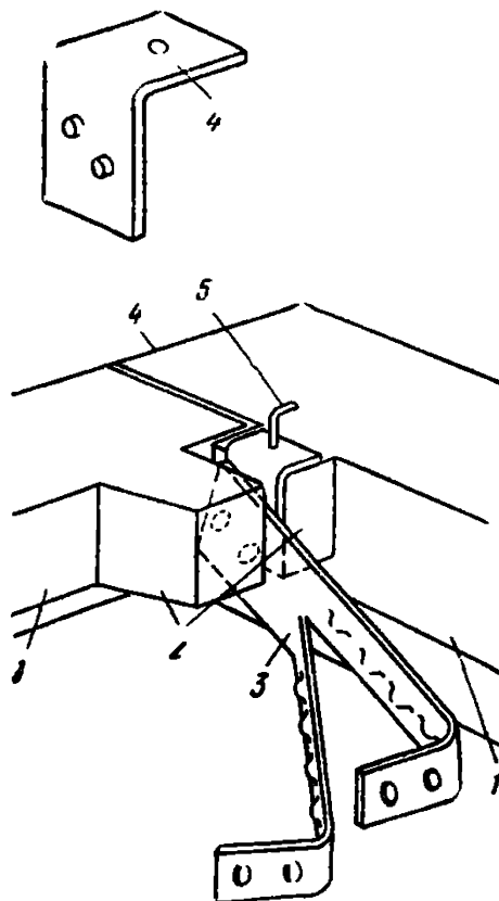
Рис. 26. Фиксация закладной детали с помощью вставки
