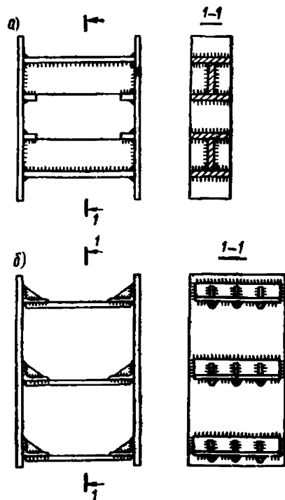
Рис. 3. Закладные детали усиленной конструкции а — с жесткими анкерами; б — с приваркой уголков
