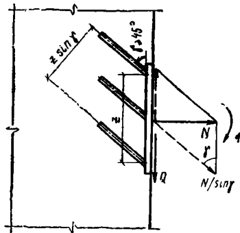
Рис. 8. Схема усилий, действующих на закладную деталь с наклонными анкерами, приваренными под слоем флюса
