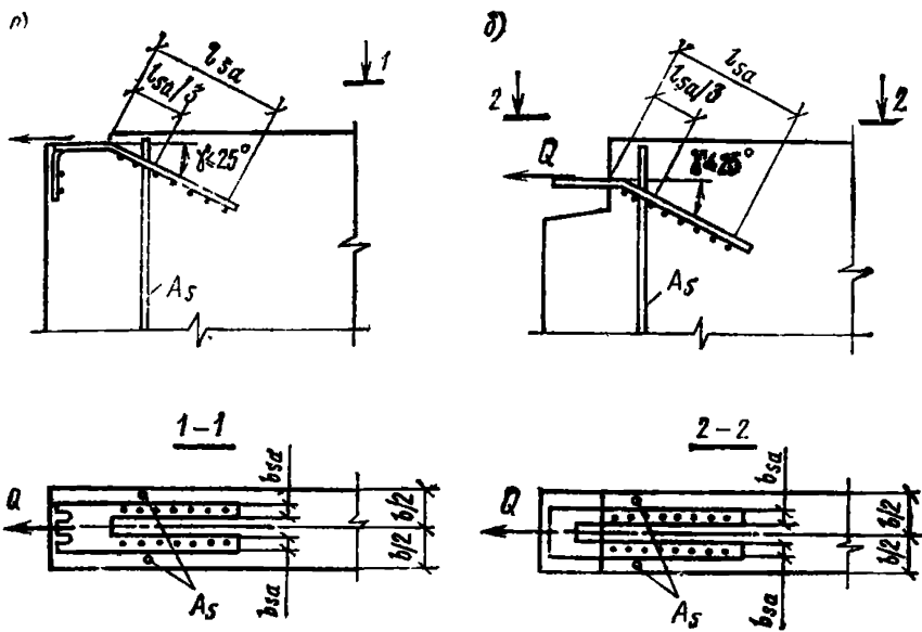
Рис. 16. Схема усилий, действующих на штампованную закладную деталь
