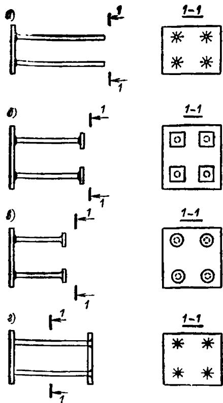
Рис. 1. Закладные детали с нормальными анкерами а — без усиления; б — с анкерными пластинами; в — с высаженными головками; г — с двумя пластинами (типа «закрытый столик»)
