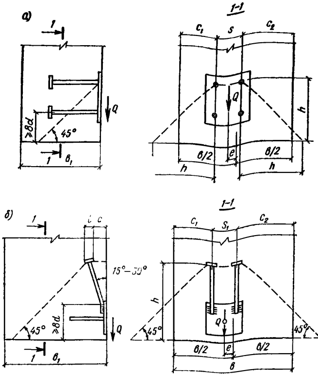
Рис. 14. Схема, принимаемая при расчете на откалывание бетона анкерами закладной детали a — нормальными; б — наклонными
