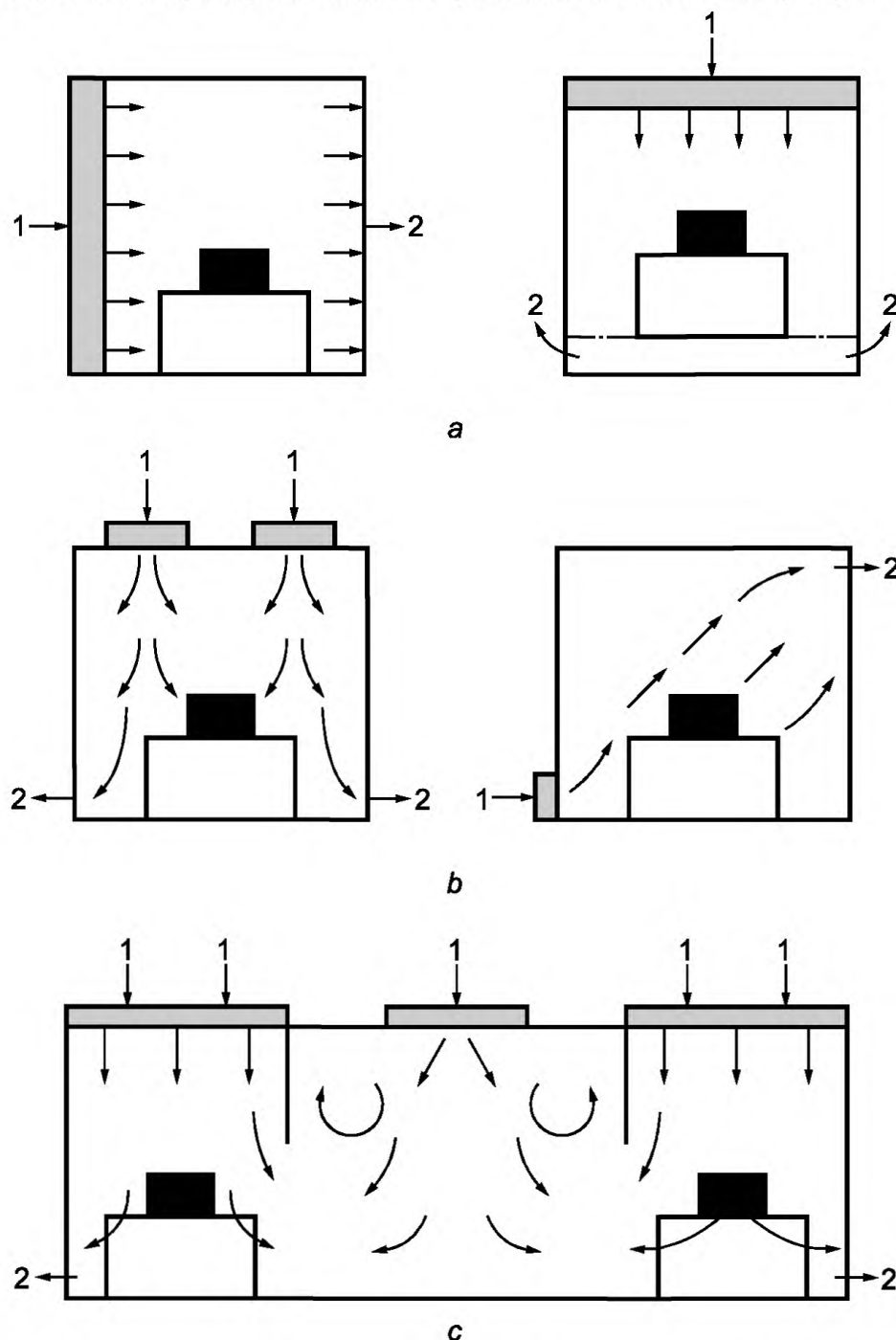
а — одна направленный поток воздуха; б — неоднаправленный поток воздуха; с — смешанный поток воздуха; 1 — приточный воздух; 2 — вытяжной воздух
