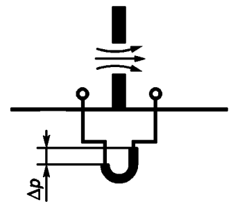
Рисунок А.7 — Принцип перепада давления
