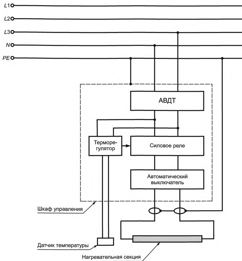
Рисунок В.2 — Принципиальная электрическая схема подключения установки распределенного электрообогрева к электрической сети с системой заземления типа TN-S
