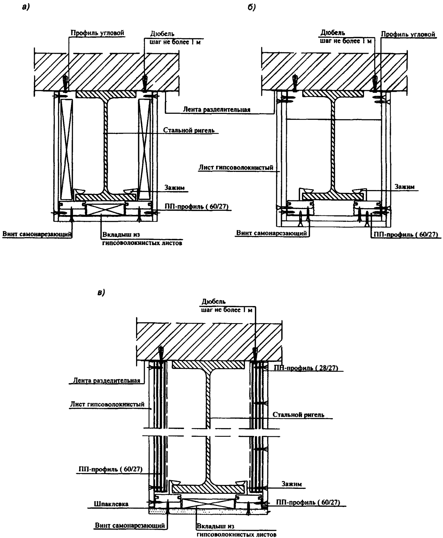
а — с металлическими профилями и одинарной обшивкой гипсоволокнистыми листами; б — то же, с двухслойной обшивкой гипсоволокнистыми листами; в — с металлическими профилями и вкладышами из гипсоволокнистых листов
