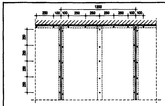
Рисунок 18 — Крепление гипсоволокнистых листов к каркасу
