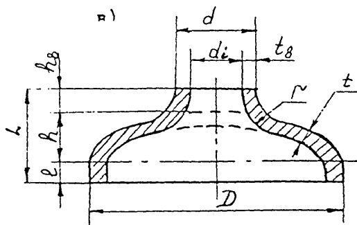
Черт.57. Эллиптические заглушки со штуцером
