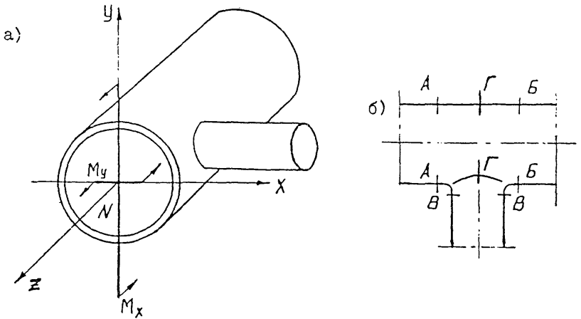
Черт. 7.2 Расчетная схема тройникового соединения
