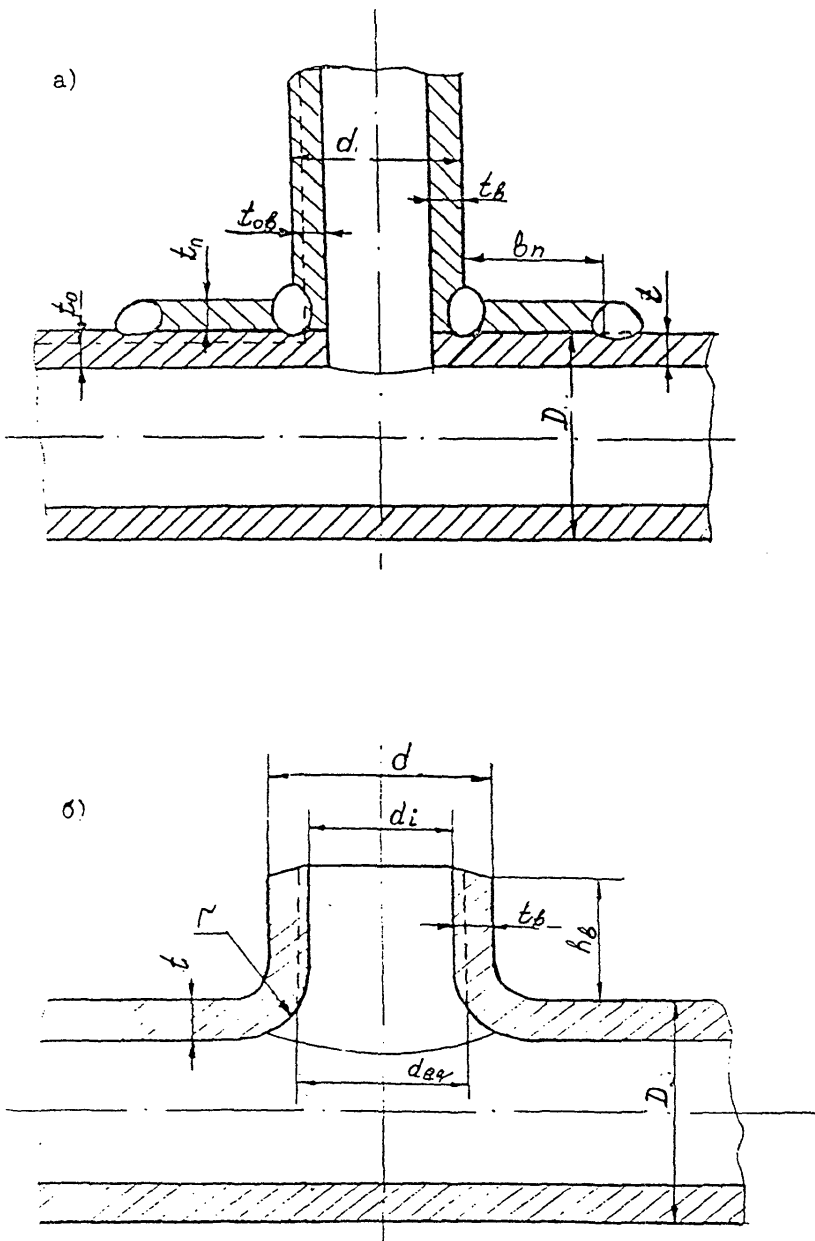
Черт. 5.3 Тройник
