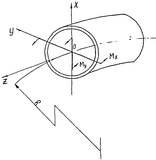
Черт. 7.1 Расчетная схема отвода
