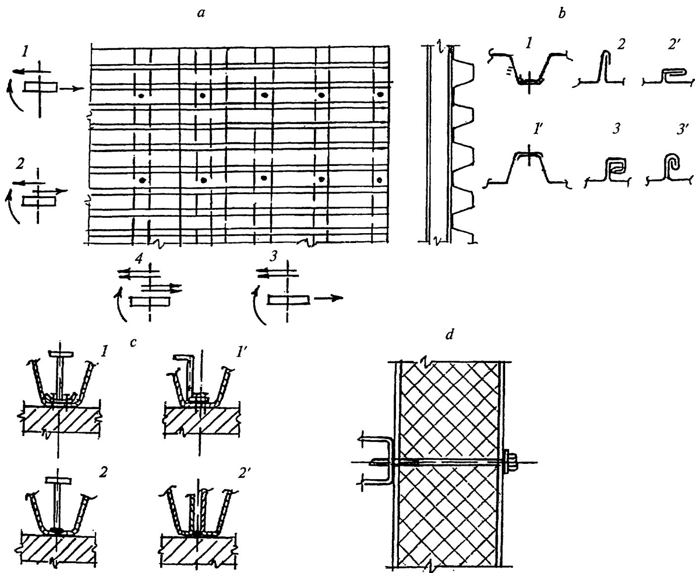
a — фрагмент конструкции покрытия со стальным профилированным настилом и схема действия сил на опорах ( 1 — соединения в среднем участке; 2 и 3 — соединения соответственно по продольным и поперечным полкам; 4 — соединения в месте пресечения продольных и поперечных полок); b — схема соединений по продольным полкам ( 1 и 1' — при расположении полок внахлест в нижнем и верхнем положениях соответственно для утепленных и холодных покрытий; 2 и 2' — простой стоячий и лежачий фальцы; 3 и 3' — варианты двойного фальца); c — сдвигоустойчивые элементы ( 1 и 1' — на высокопрочных дубелях; 2 — на контактной сварке; 2' — на дуговой сварке); d — фрагмент трехслойной стеновой панели на самосверлящем винте
