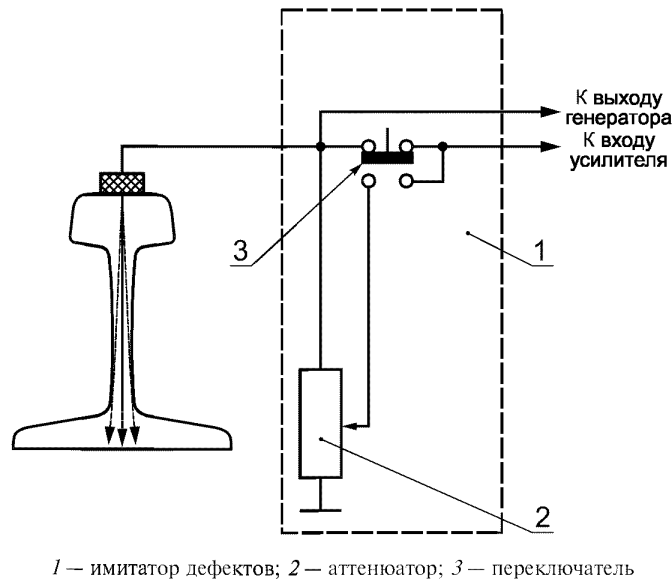
Рисунок 1 — Схема устройства для измерения условной чувствительности
