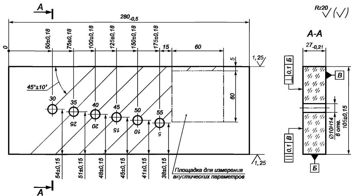
Рисунок 2 — Стандартный образец СО-1Р
