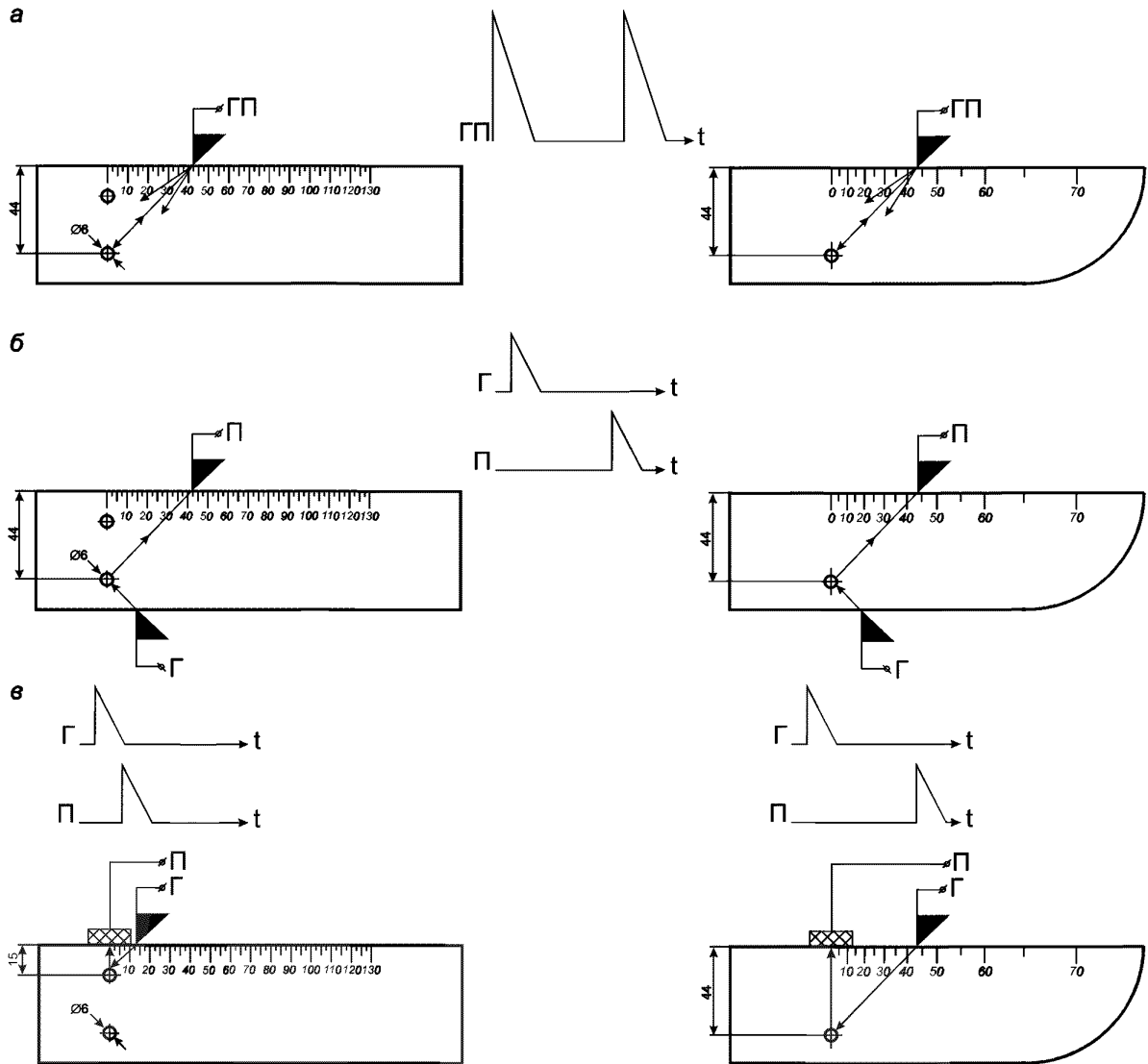
Рисунок 5 — Схема расположения преобразователей на стандартном образце СО-2Р (СО-3Р) при измерении (настройке) условной чувствительности при контроле: a — эхо-методом, б — зеркальным методом, в — дельта-методом
