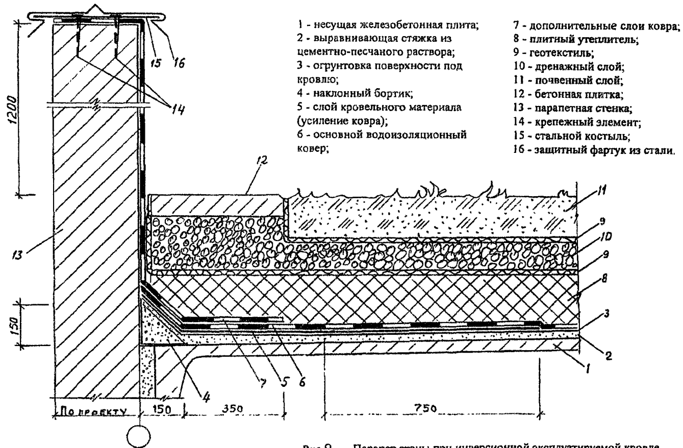
Рис.9 Парпет стены при инверсионной эксплуатируемой кровле.
