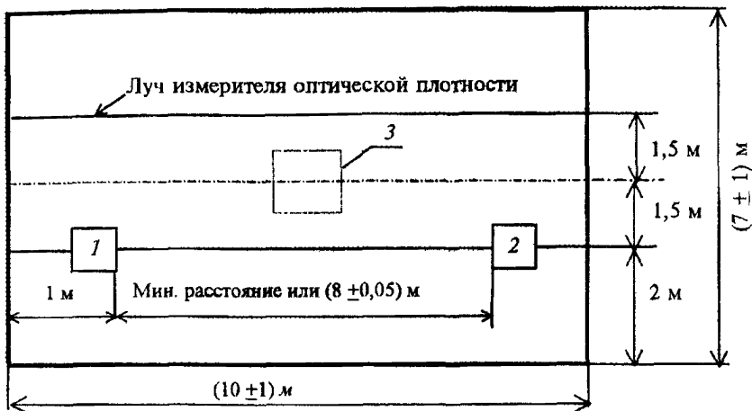
Схема расположения ИПДЛ и контрольно-измерительной аппаратуры при проведении огневых испытаний:
