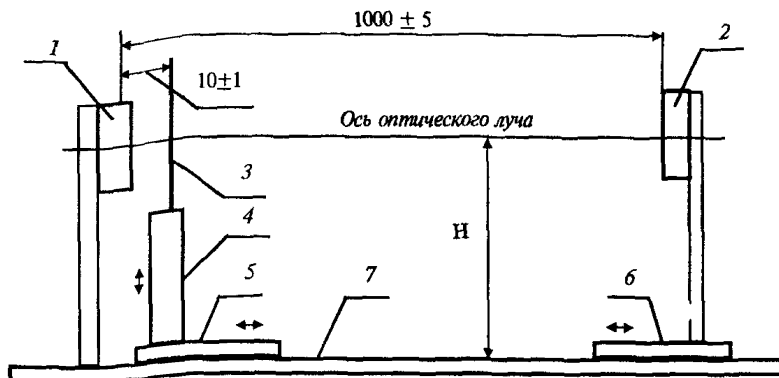
Рис. 1. Схема расположения элементов ИПДЛ и аттенюатора (вариант 1 - передатчик и приемник):
