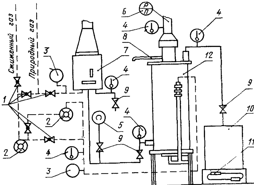
1—пробковый кран; 2—газовый счетчик; 3—мановакуумметр; 4—термометр; 5—манометр; 6—тягианометр; 7—аппарат водонагревательный проточный; 8—пробоотборник; 9—вентиль; 10—сосуд для воды; 11—весы; 12—аппарат водонагревательный емкостной.
