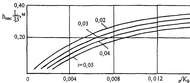
Рис. 5.2. Номограмма для расчета дренирующего слоя из крупных песков с коэффициентом фильтрации более 10 м/сут L – длина пути фильтрации в м, равная B при односкатном профиле и 0,5B при двухскатном; i – поперечный уклон низа дренирующего слоя; K_{\phi} – коэффициент фильтрации, м/сут
