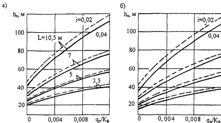
Рис. 5.4. Номограмма для расчета дренающего слоя в конструкции с прикромочным дренажем: а – мелкий песок; б – песок средней крупности
