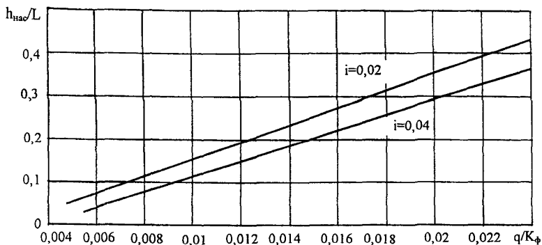
Рис. 5.1. Номограмма для расчета толщины h_{\text{нас}} дренирующего слоя из песков мелкой и средней крупности, а также крупнозернистых с коэффициентом фильтрации менее 10 м/сут. При односкатном поперечном профиле q' = q_p B [м 3 /м]; при двухскатном поперечном профиле q' = 0,5q_p B [м 3 /м]; B – ширина проезжей части, м; L – длина пути фильтрации, равный B при односкатном профиле и 0,5B при двухскатном
