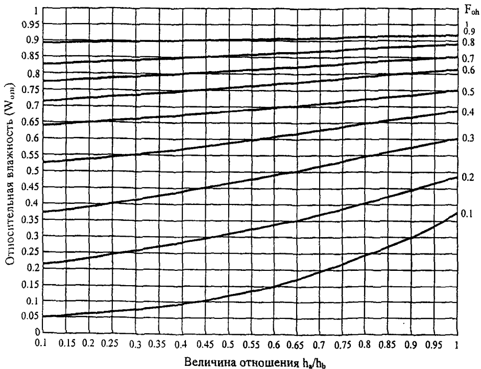
Рис. П.7.2. Номограмма для W_{om} при значениях F_{oh} от 0,1 до 1
