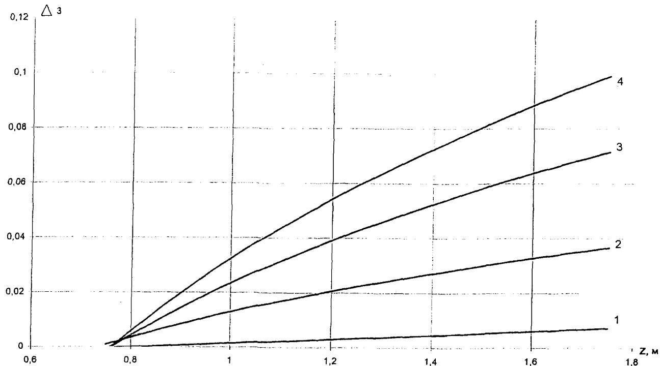
Рис. П.2.1. Графики для определения поправки на влияние суммарной толщины стабильных слоев одежды: 1 - для исходной* относительной влажности 0,75 Вт; 2 - то же, для 0,80 Вт; 3 - то же, для 0,85 Вт; 4 - то же, для 0,90 Вт.
