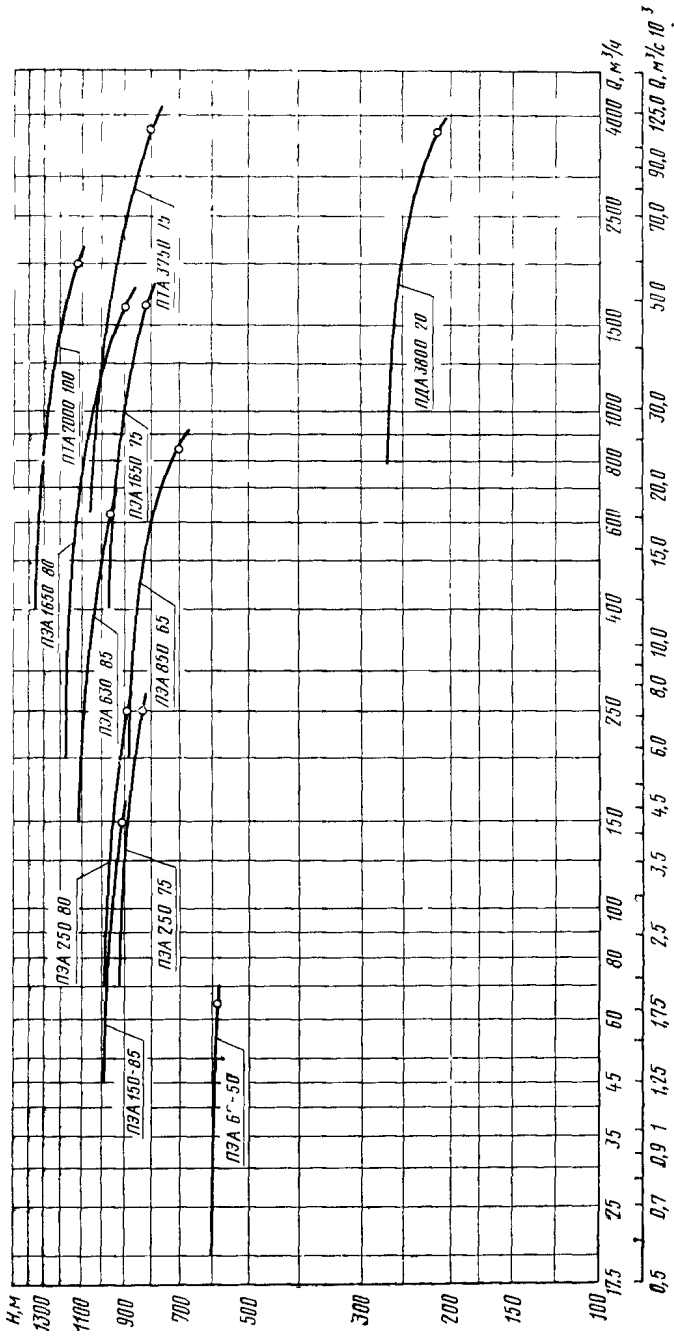
Рабочие части характеристик Q \rightarrow H
