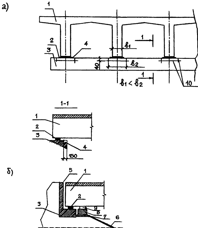
Рис. 5.4. Расположение домкратов на устое в бездиафрагменном пролетном строении с устройством ниши (а) и с использованием сваи (б):
