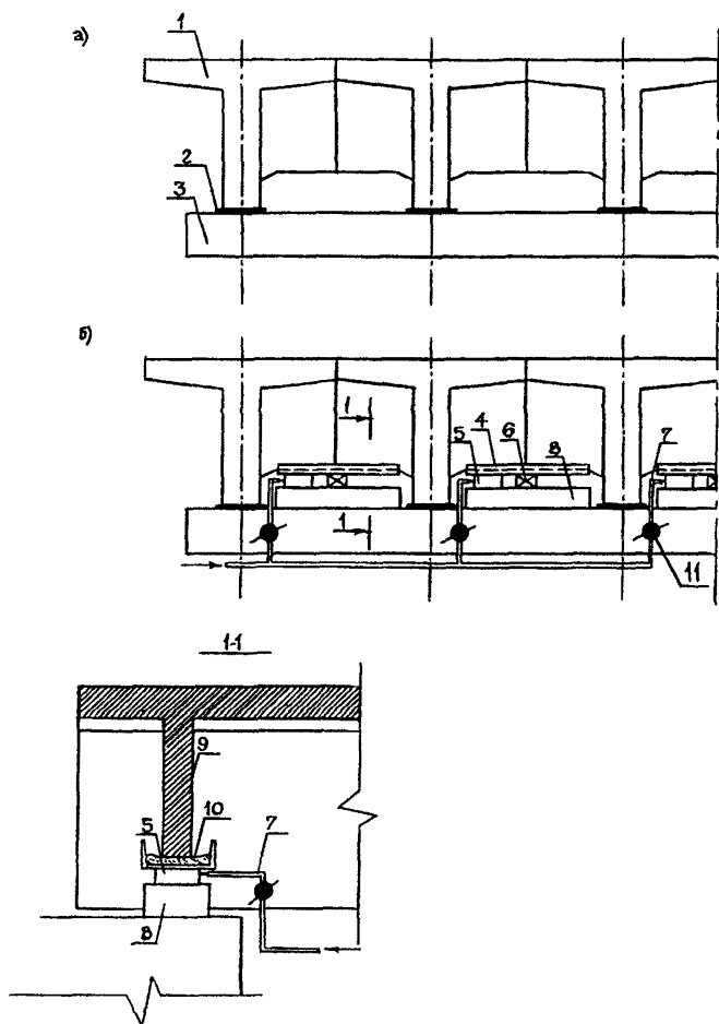
Рис. 5.3. Схема подготовки диафрагм:
