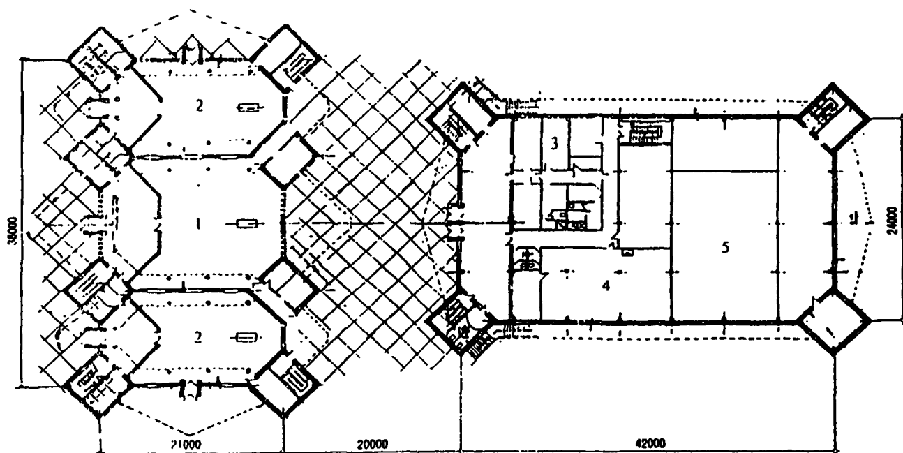
План на отм. 3,300
