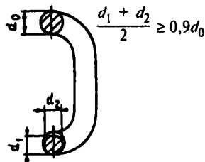
Рис. 2. Уменьшение диаметра сечения звена цепи:
