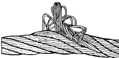
Рис. 11. Выдавливание сердечника
