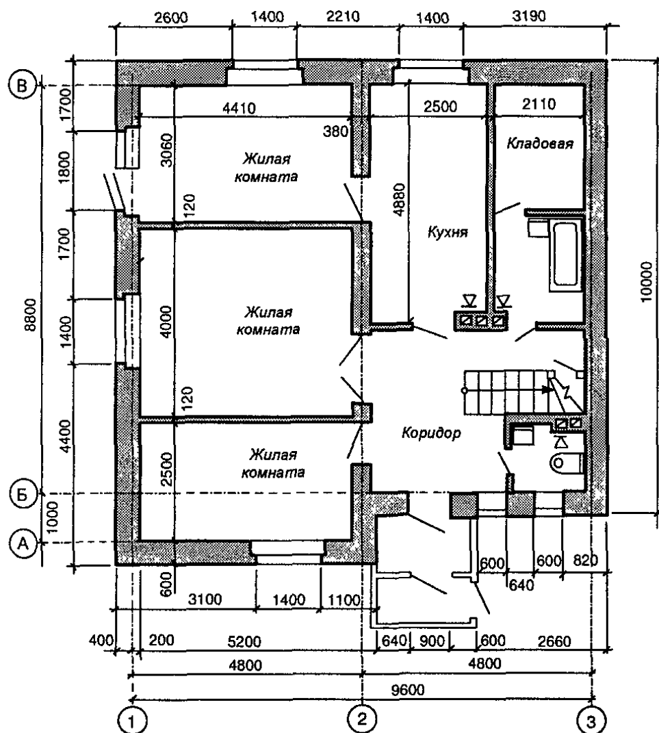
Рис. В. Схематичные планы этажей и разрез дома
