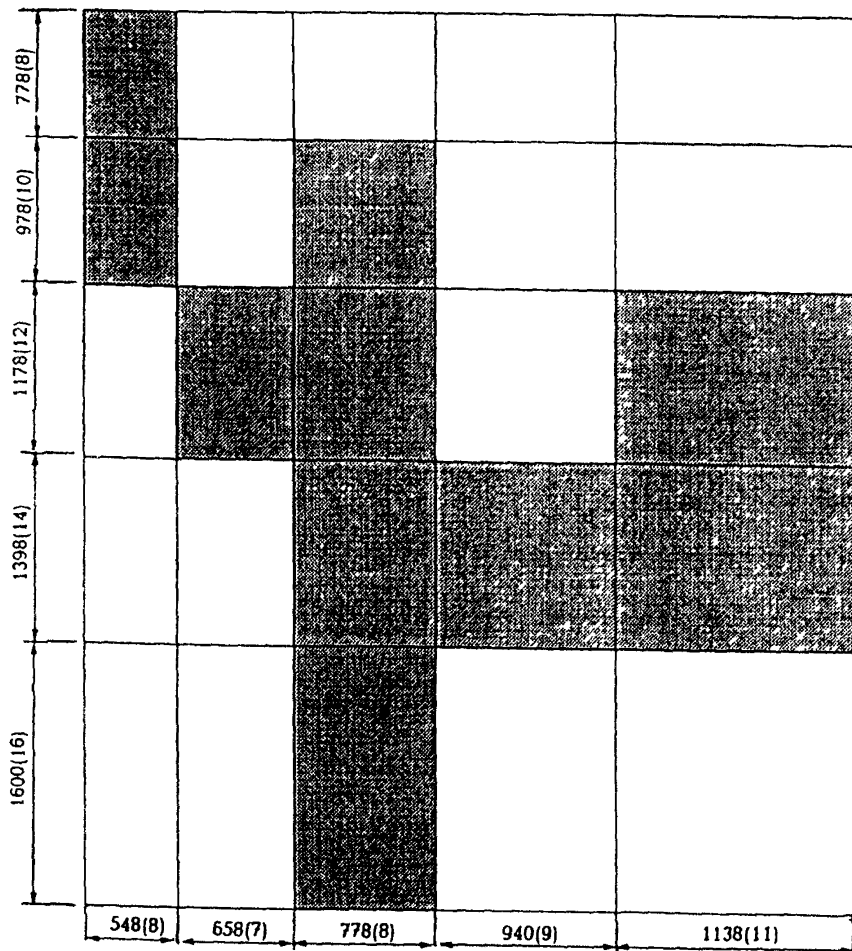
Рисунок 2 — Рекомендуемые габаритные размеры мансардных оконных блоков (мм)
