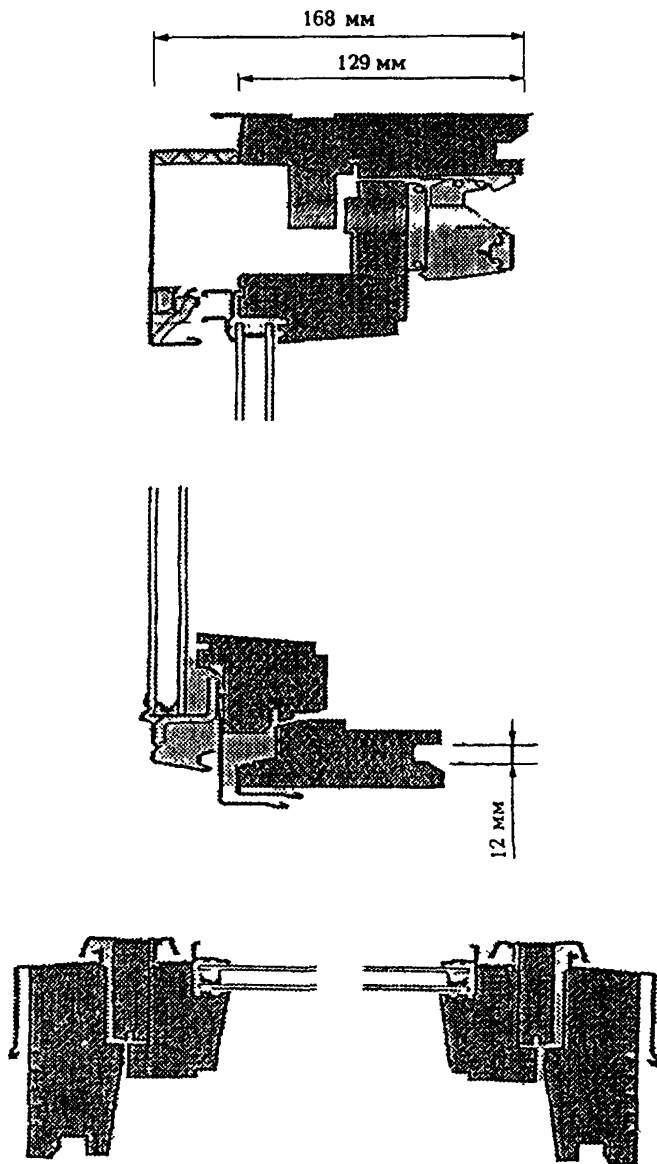
Рисунок 3 — Пример конструктивного решения мансардного оконного блока
