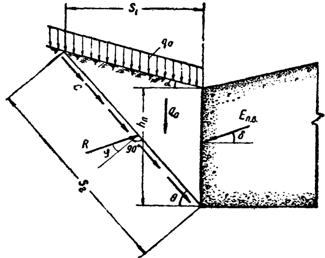
Рис. 13. К расчету пассивного давления с выпором при связных грунтах
