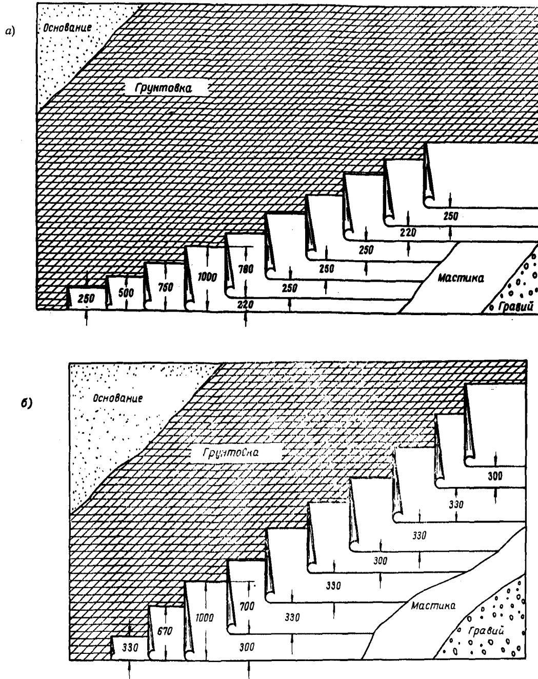
Рис. 1. Пример технологии устройства кровель а—устройство четырехслойной кровли; б—устройство трехслойной кровли
