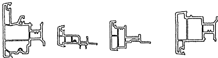
Сечения профилей шульпов
