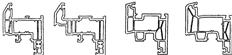
Сечения профилей створок
