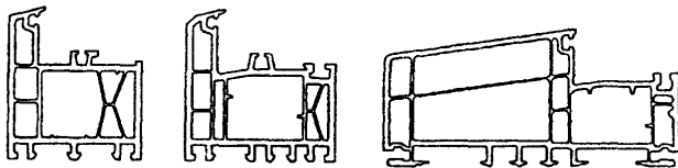
Сечения профилей коробок
