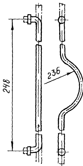
Рис.33. Антивибрационный крововой зажим ЗАК-10-І: І - провод; 2 - изолятор; 3 - скоба; 4 - захватывающая скоба
