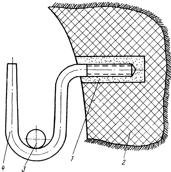
Рис.14. Крепление крюков в тоннелях: 1 - алебастр; 2 - стенка тоннеля; 3 - кабель связи; 4 - крюк (скоба)
