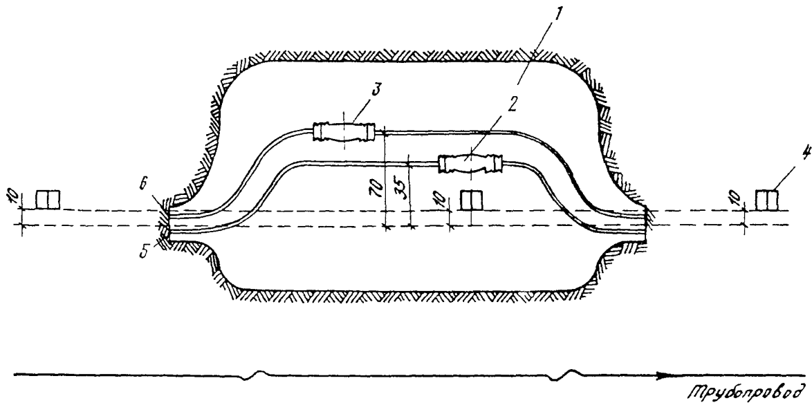
Рис.16. Установка измерного столбика у муфт на двухкабельной линии связки: 1 - котлован; 2 - муфта № 1; 3 - муфта № 2; 4 - измерный столбик; 5 - кабель № 1; 6 - кабель № 2
