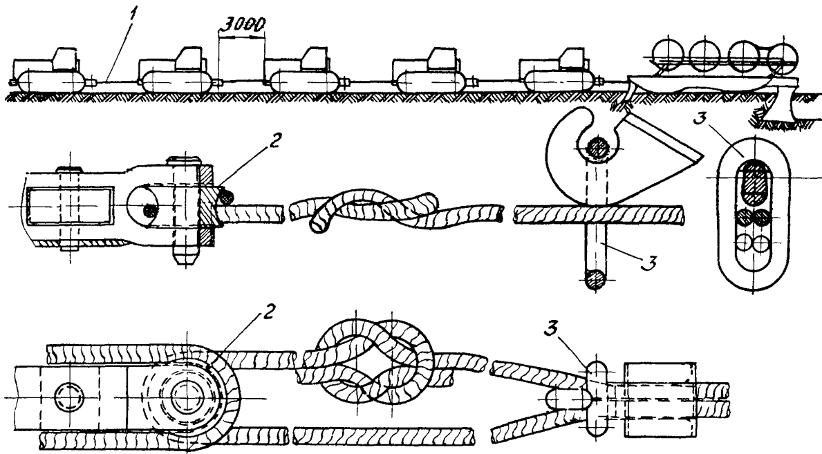
Рис.2. Сцепка тракторов тросами: 1 - трос диаметром 36 мм; 2 - ролик форкопа; 3 - петля крюка
