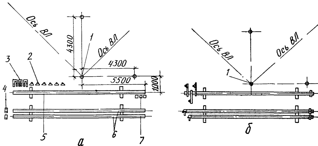
Рис.26. Сборка железобетонных опор на пикете:
