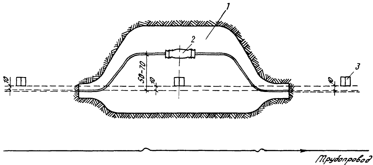
Рис.15. Установка измерного столбика у муфты на однокабельной линии связи: 1 - котлован; 2 - муфта; 3 - измерный столбик
