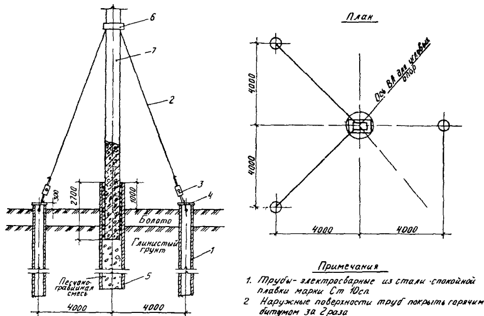
Рис. 30. Закрепление анкерно-угловых опор на болотах и пучинистых грунтах:
