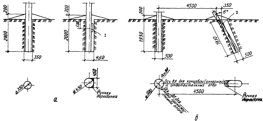
Рис.27. Разработка котлованов: а - под промежуточные опоры; б - под сложные опоры; I - ригель; 2 - подкос
