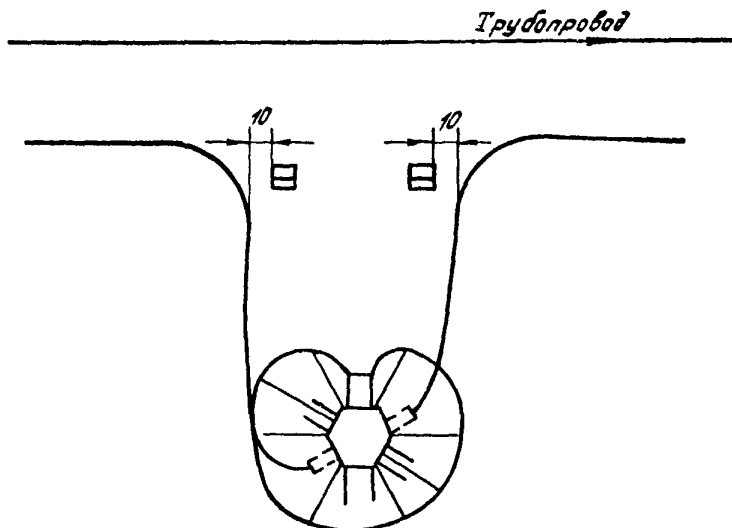
Рис.21. Установка дополнительных столбиков у НУПа
