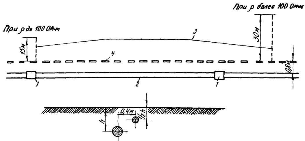
Рис.24. Схема прокладки одного защитного провода (трасса): 1 - муфта; 2 - кабель; 3 - лучевой заземлитель; 4 - защитный провод
