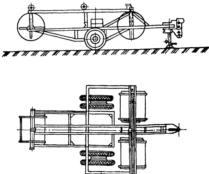
Рис. 32. Одноосная трехбарабанная саморазгружающаяся раскаточная тележка грузоподъемностью 3 т; габариты: 4550х2790х2100 мм
