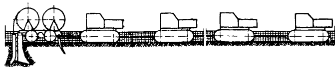
Рис.3. Обычная сцепка при работе на твердых грунтах и на болотах глубиной до I м с твердым дном
