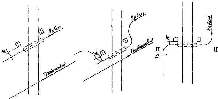
Рис.20. Установка замерных столбиков на переходах кабеля автомобильных и железных дорог в защитных трубах
