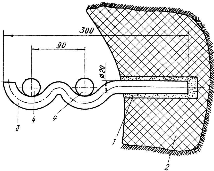
Рис.13. Крепление скоб в тоннелях:
