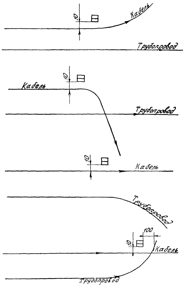
Рис.18. Столбик дополнительный в местах отхода кабеля от трубопровода
