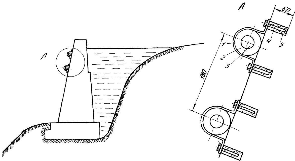
Рис.II. Схема прокладки кабеля по подпорной стене:
