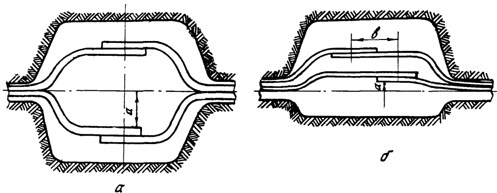
Рис.22. Выкладка кабелей в котловане: а - по обе стороны от оси траншей; б - по одну сторону от оси траншей
