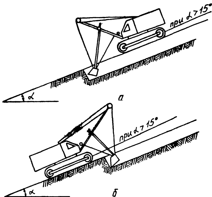
Рис.8. Схема работы на уклоне одноковшового экскаватора: а - с прямой лопатой; б - с обратной лопатой
