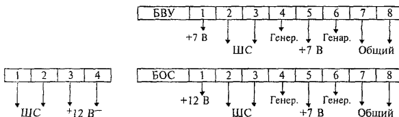
Рисунок 3.19 - "Стекло-1"
