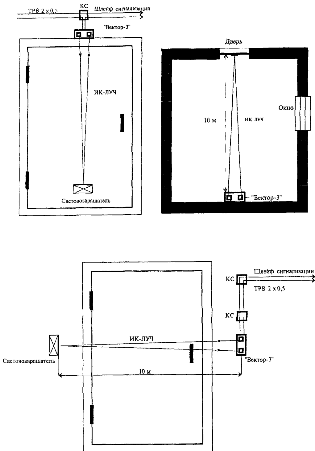
Рисунок 6 14 - Блокировка дверей (ворот) на открывание извещателями активными линейными опико-электронными
