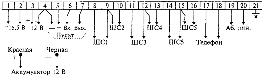
Рисунок 4.26 - "Vista-101"
