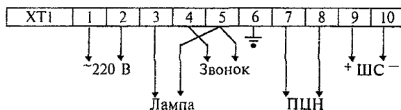
Рисунок 4.8 - "Сигнал-31"
