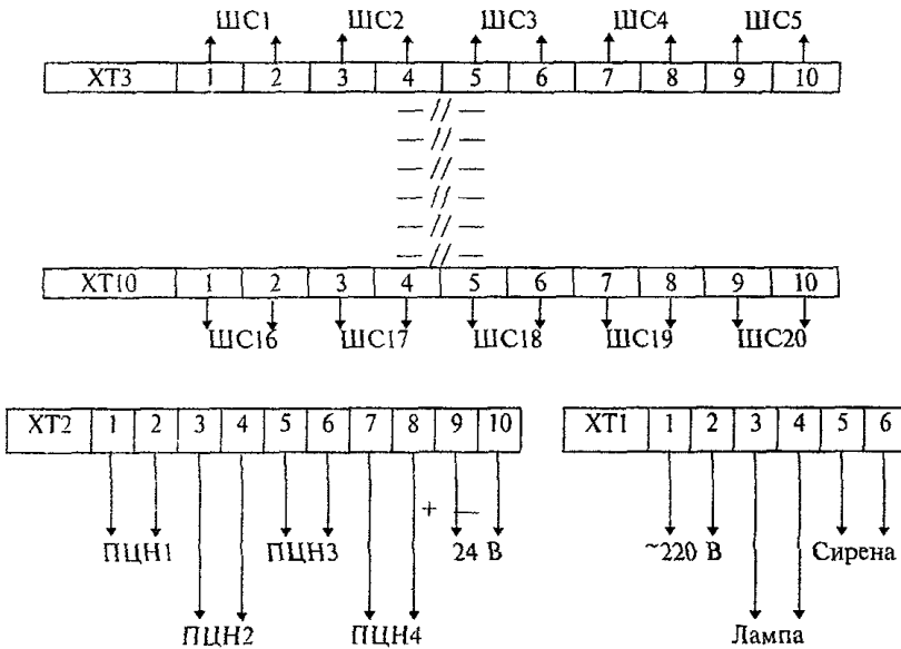
Рисунок 4.25 - "Пульсар"
