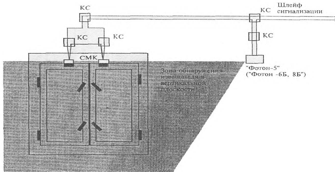
Рисунок 6.7 - Блокировка окна на открывание и проникновение извещателями магнитоконтактными и пассивными оптико-электронными с зоной обнаружения типа "занавес"
