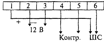
Рисунок 3.30 - "Тюльпан-3"
