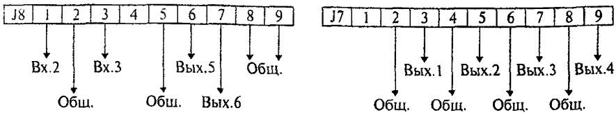
Рисунок 4.29 - "Vista-501"
