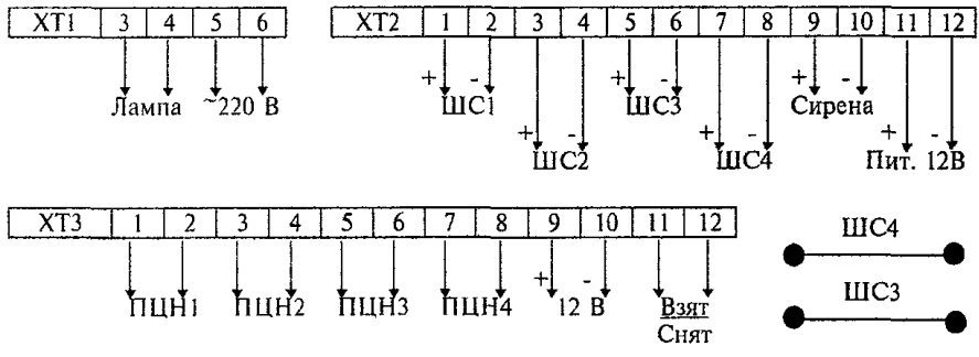
Рисунок 4.17 - "Сигнал-ВК-4"
