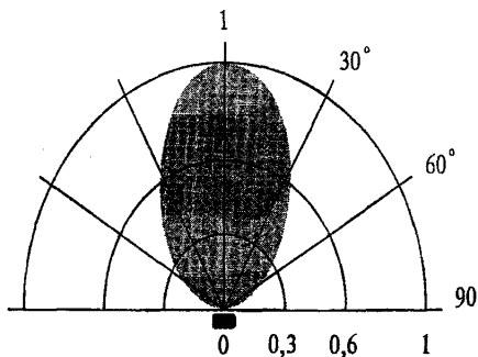
Рисунок 3.50 - Извещатель "Аргус-3"
