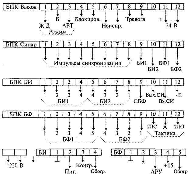
Рисунок 3.25 - "Рубеж-3М"
