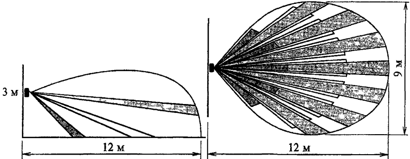
Рисунок 3 57 - Извещатель “Сокол-1”
