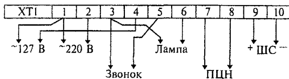
Рисунок 4.7 - "Сигнал-3М-1"
