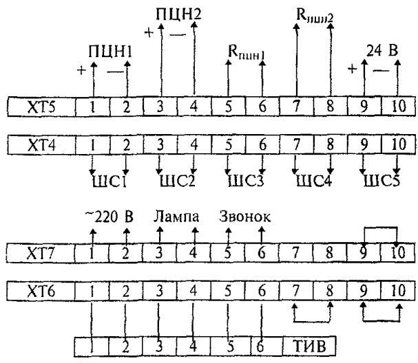
Рисунок 4.19 - "Квинта"
