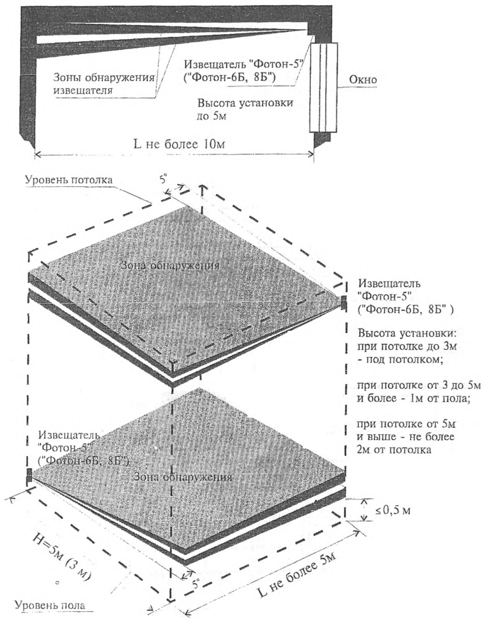
Рисунок 6.24 - Блокировка стен, потолка и пола на проникновение извещателями пассивными оптико-электронными с зоной обнаружения типа " занавес ".
