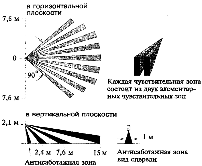
Рисунок 3.47 - Извещатель "9981"
