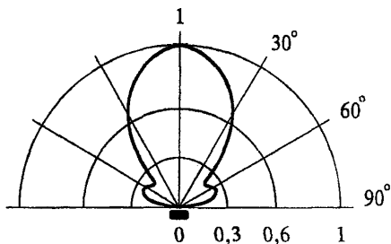
Рисунок 3.49 - Извещатель "Аргус-2"
