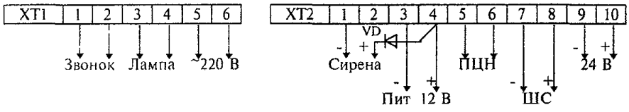
Рисунок 4.16 - "Сигнал-ВК", "Сигнал-ВК-Р"
