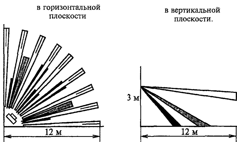
Рисунок 3.42 - Извещатель "Фотон-4"
