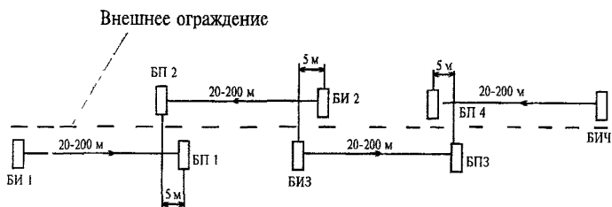
Рисунок 6.47 - Размещение извещателей "Радий-1" ("Радий-2") при блокировке замкнутого периметра
