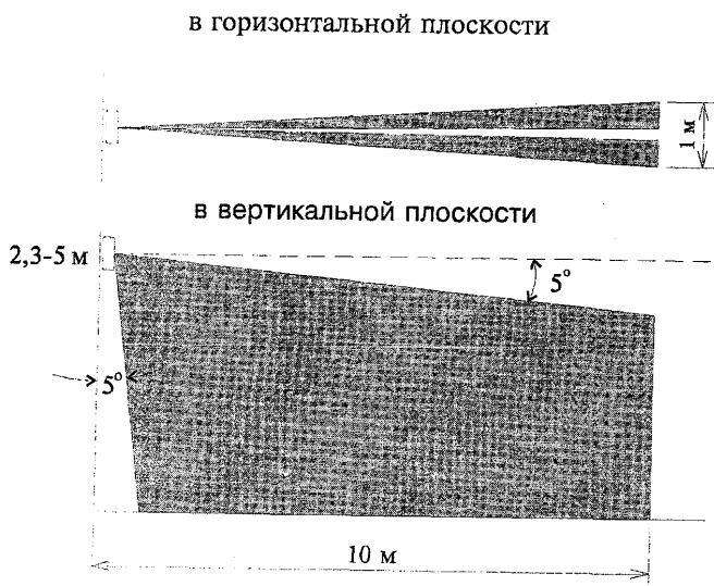
Рисунок 3.43 - Извещатель "Фотон-5"
