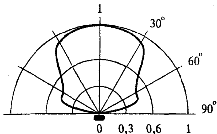
Рисунок 3.49 - Извещатель "Аргус-2"
