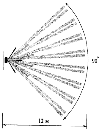
Рисунок 3.44 - Извещатели "Фотон-6", "Фотон-8" (объемная зона)
