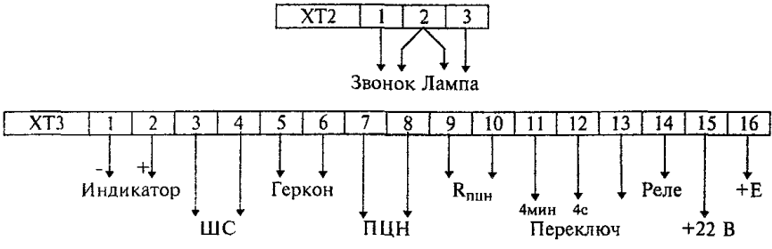
Рисунок 4.15 - "Сигнал-45"
