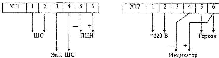
Рисунок 4.13 - "Сигнал-41М"
