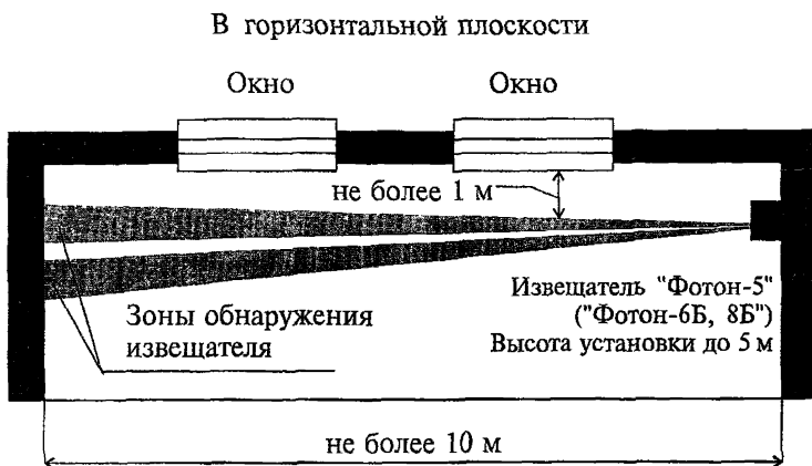
Рисунок 6.6 - Блокировка оконных проемов на проникновение извещателями пассивными оптико-электронными с зоной обнаружения типа "занавес"
