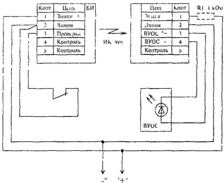
Рисунок 7.6 - Извещатель типа ИП 212-5 “ДИП-3”
