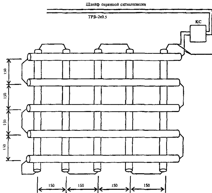
Рисунок 6.22 - Блокировка фальшрешетки воздуховода проводом
