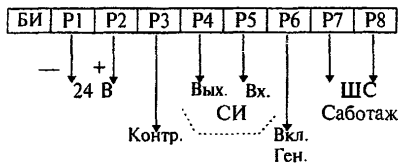
Рисунок 3.37 - “Вектор-СПЭК”
