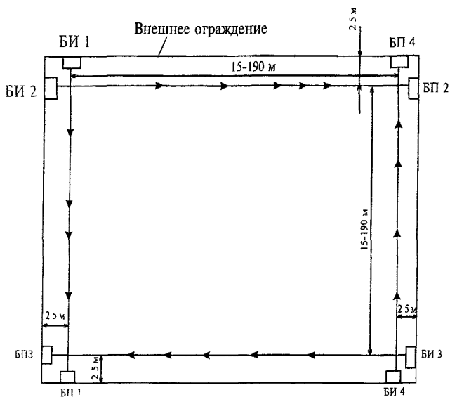
Рисунок 6.47 - Размещение извещателей "Радий-1" ("Радий-2") при блокировке замкнутого периметра
