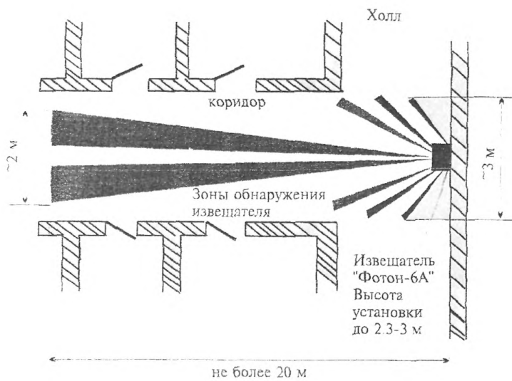
Рисунок 6.38 - Блокировка коридора и холла извещателями пассивными опико-электронными с линейной зоной обнаружения
