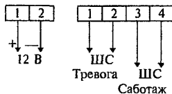
Рисунок 3.28 - "Фотон-СК"
