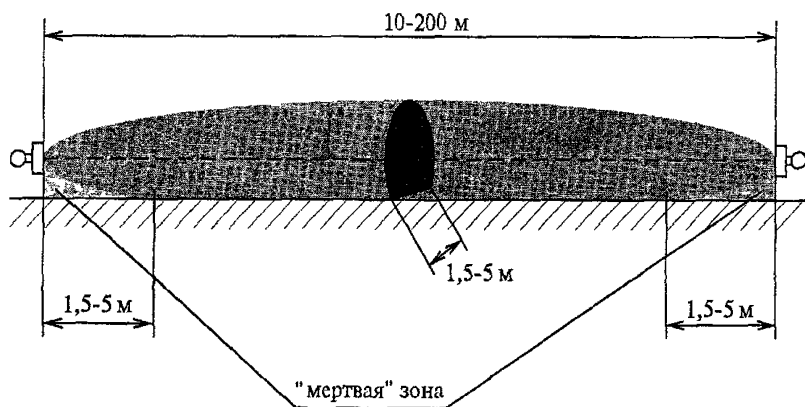
Рисунок 3 54 - Извещатель "Радий-2"
