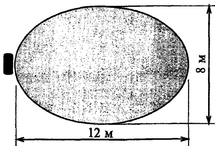
Рисунок 3.51 - Извещатель "Волна-5"
