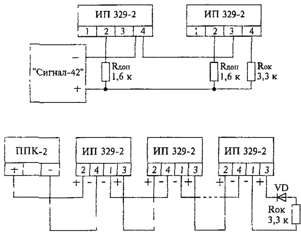
Рисунок 7.8 - Извещатель ИП 329-2 “Аметист”
