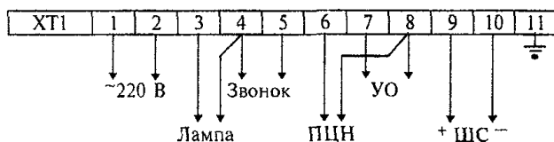
Рисунок 4.9 - "Сигнал-37А", "Сигнал-37М", "Сигнал-37Ю"
