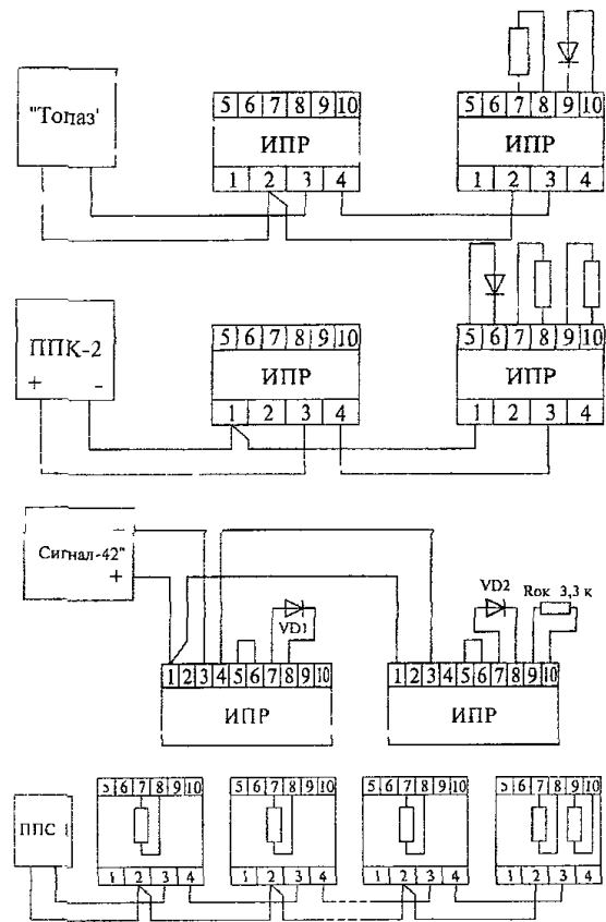
Рисунок 7.9 - Извещатель ИПР
