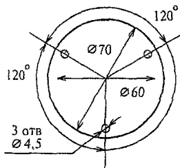
Рисунок 3 6 - "Эхо-2"
