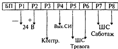
Рисунок 3.37 - “Вектор-СПЭК”
