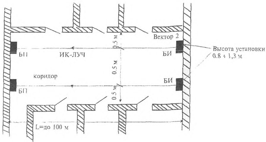
Рисунок 6.37 - Блокировка коридора извещателями линейными активными опико-электронными
