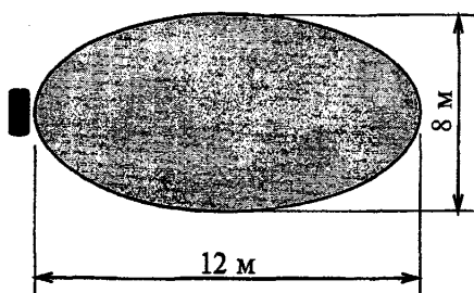
Рисунок 3.51 - Извещатель "Волна-5"
