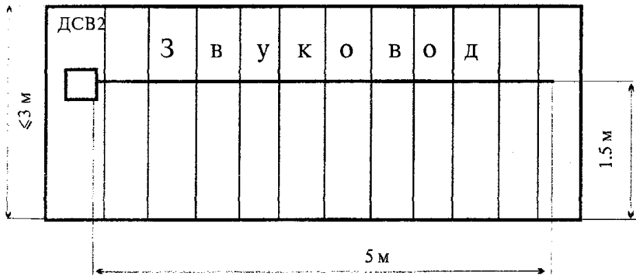
Рисунок 6.25 - Блокировка стен, потолка и пола на пролом извещателем поверхностным "Грань-2"
