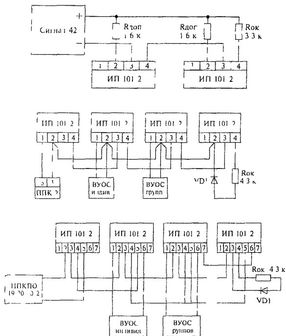
Рисунок 7 4 - Извещатель ИП 101-2
