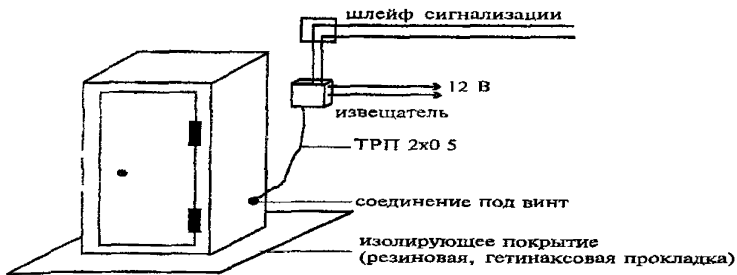
Рисунок 6 31 - Блокировка сейфа извещателем емкостным "Пик"
