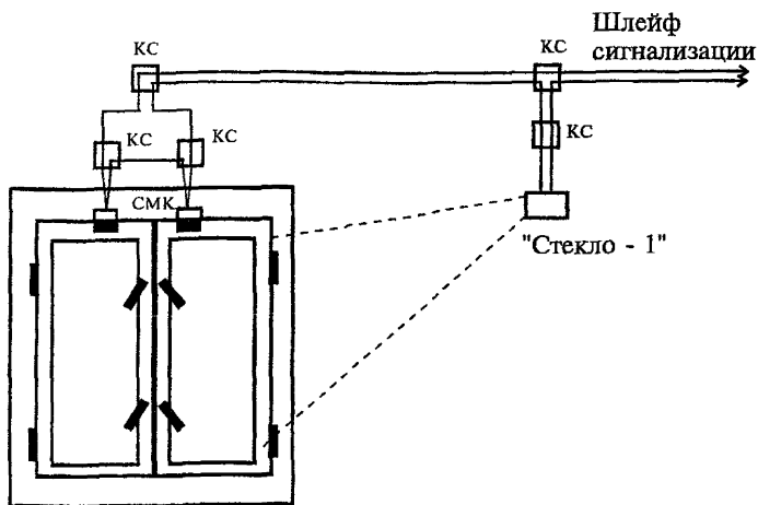
Рисунок 6.5 - Блокировка окна на открывание и разрушение извещателями "Стекло-1" и магнитоконтактными
