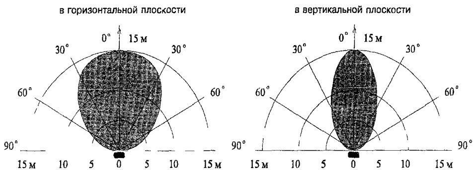
Рисунок 3 52 - Извещатель "Тюльпан-3"
