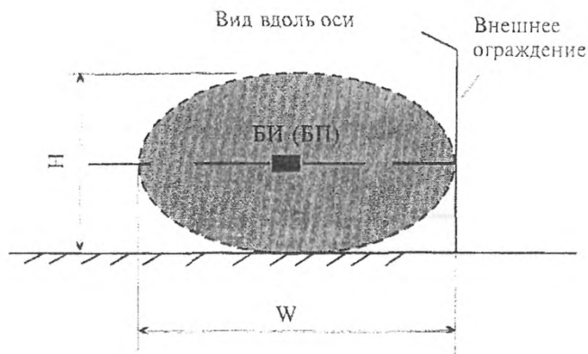
Рисунок 6.46 - Блокировка внешнего ограждения извещателем радиоволновым "Радий-1" ("Радий-2")
