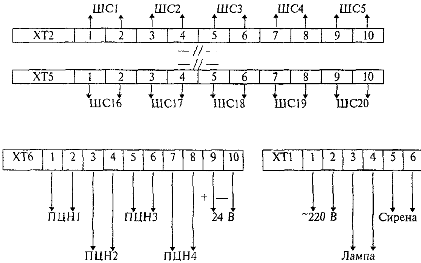
Рисунок 4.23 - "Рубин-6"
