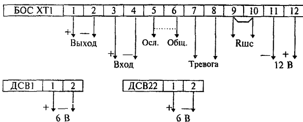
Рисунок 3.15 - "Грань-2"
