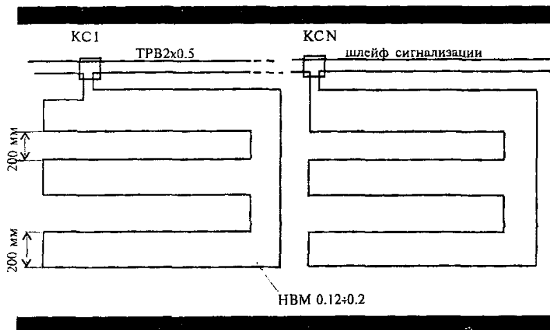
Рисунок 6.22 - Блокировка фальшрешетки воздуховода проводом
