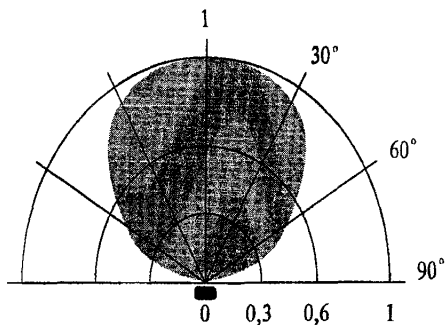
Рисунок 3.50 - Извещатель "Аргус-3"
