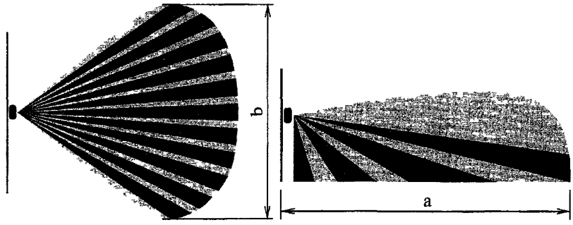
Рисунок 3 58 - Извещатели “DT4351T”, “DT4501T”, “DT4201T”
