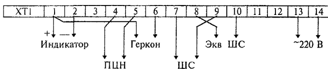
Рисунок 4.12 - "Сигнал-41"
