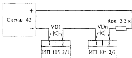
Рисунок 7 5 - Извещатель ИП 105-2/1
