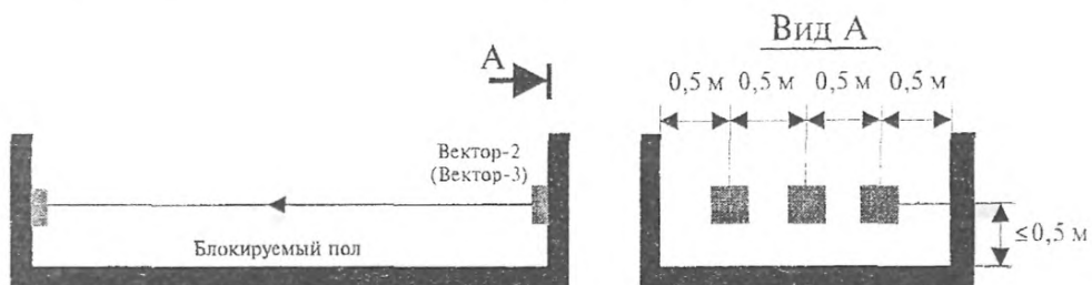
Рисунок 6.27 - Блокировка стен, потолка и пола на проникновение извещателями активными линейными оптико-электронными
