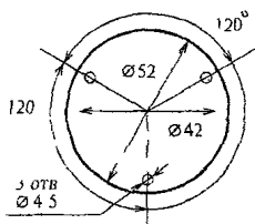
Рисунок 3 7 - "Эхо-3"
