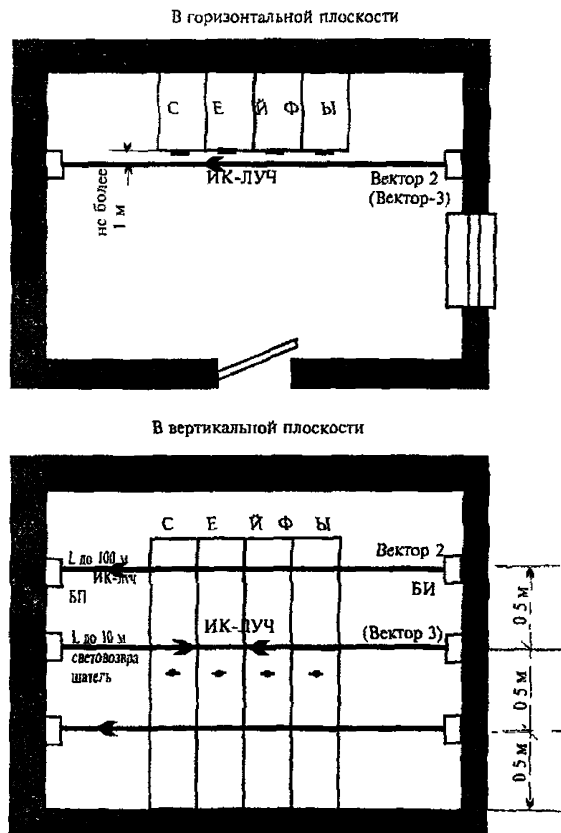
Рисунок 6.35 - Блокировка сейфов (предметов) извещателями линейными активными оптико-электронными
