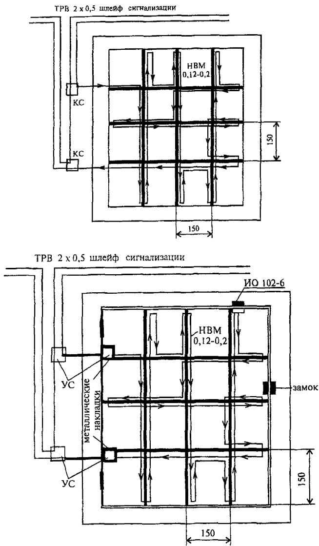
Рисунок 6.21 - Блокировка оконных решеток, решеток воздухопроводов и решетчатых дверей проводом
