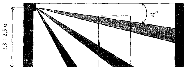
Рисунок 6.18 - Блокировка двери на проникновение объемным оптико-электронным извещателем
