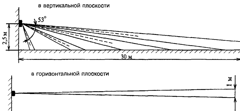
Рисунок 3.41 - Извещатель "Фотон-2"
