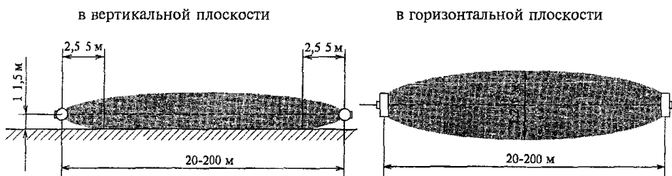
Рисунок 3 53 - Извещатель "Радий-1"
