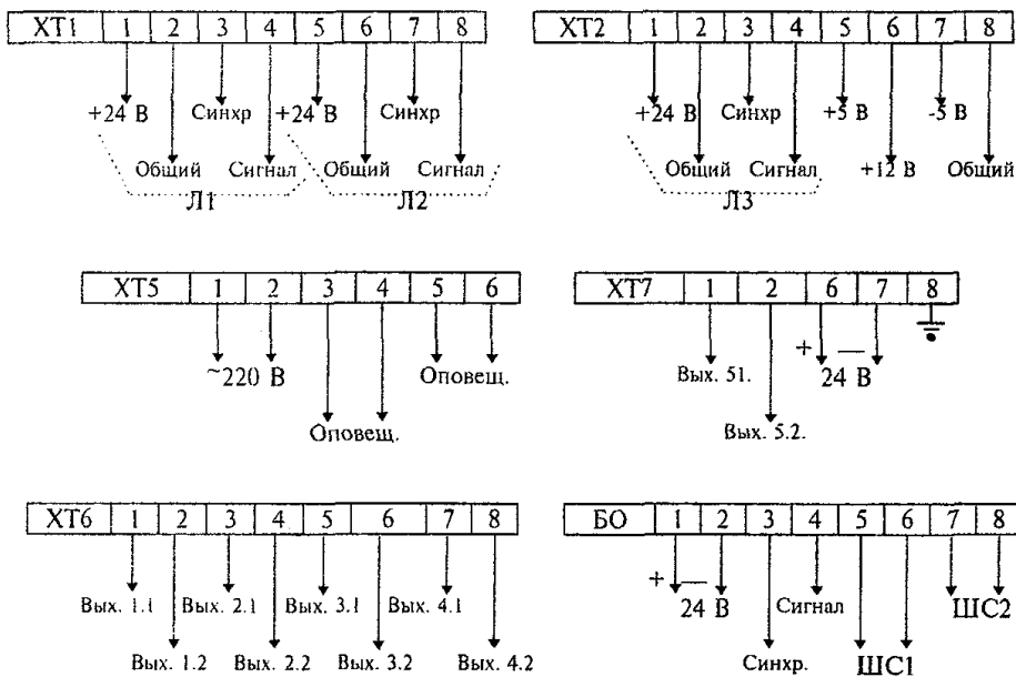
Рисунок 4. 27 - "Буг"
