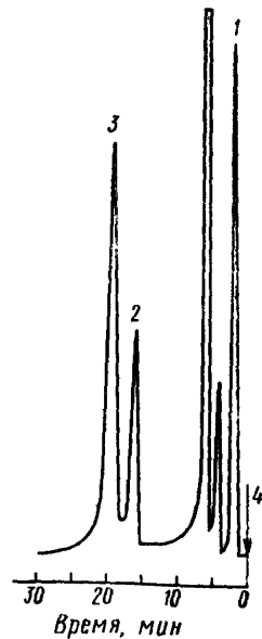
Хроматограмма фенолоформальдегидных смол, содержащих ацетон
