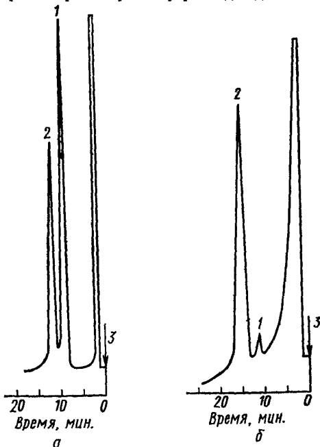
Хроматограмма фенолоформальдегидных смол
