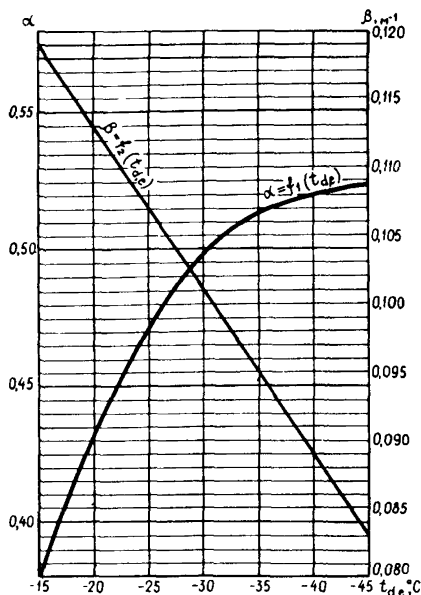
Черт. 9. Графики зависимости коэффициентов \alpha и \beta от t_{d,e}
