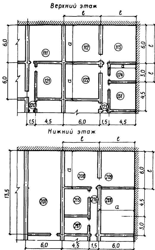
Черт. 10. Фрагменты планов этажей
