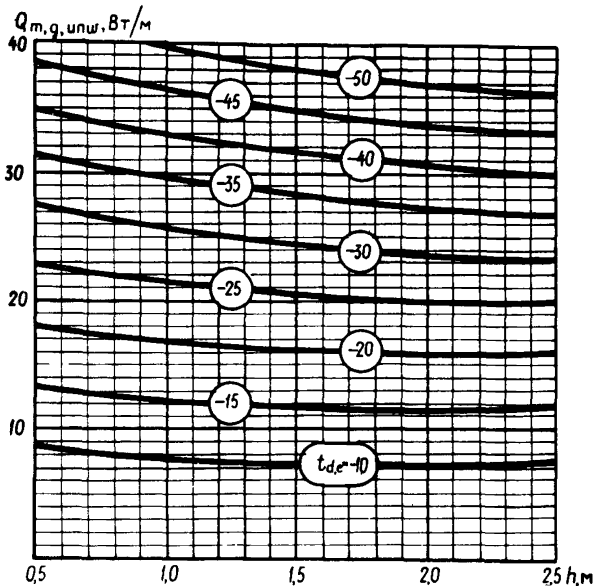
Черт. 7. Графики зависимости Q_{m,g,upw} от h и t_{d,e}
