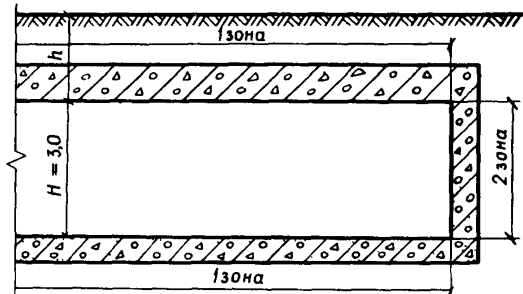
Черт. 1. Разбивка на зоны ограждений одноэтажного сооружения
