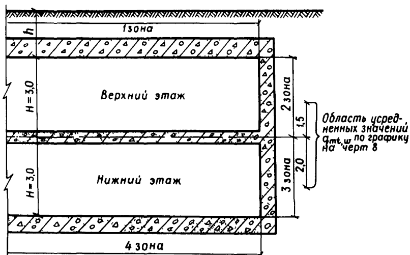
Черт. 4. Разбивка на зоны ограждений двухэтажного сооружения
