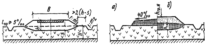
Рис. 11. Типовая схема земляного полотна, возведенного на поверхности слабой толщи
