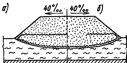
Рис. 23. Конструкция насыпи
