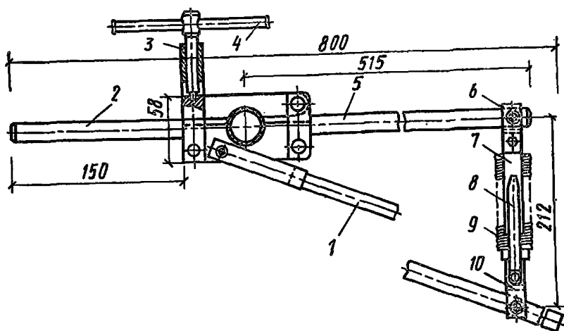
Рис. 5. Динамометрическое устройство
