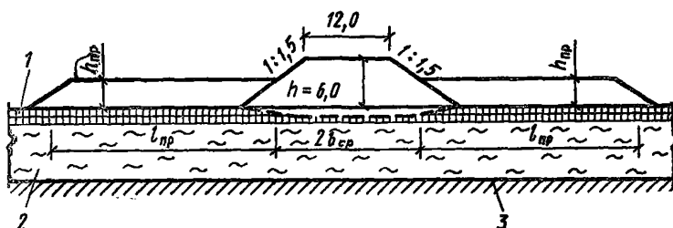
Рис. 1. Расчетный поперечник
