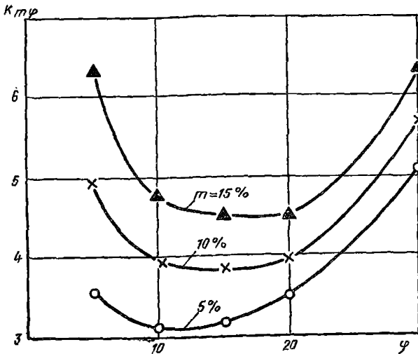
Рис. 9. График зависимости k_{\text{мф}} = f(\varphi) при различных значениях m
