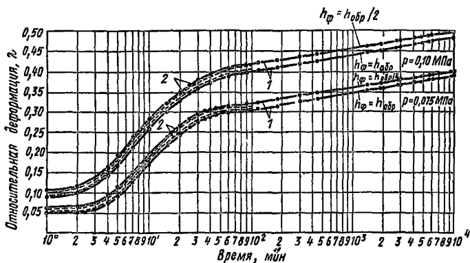
Рис. 11. Построение исправленных кривых консолидации
