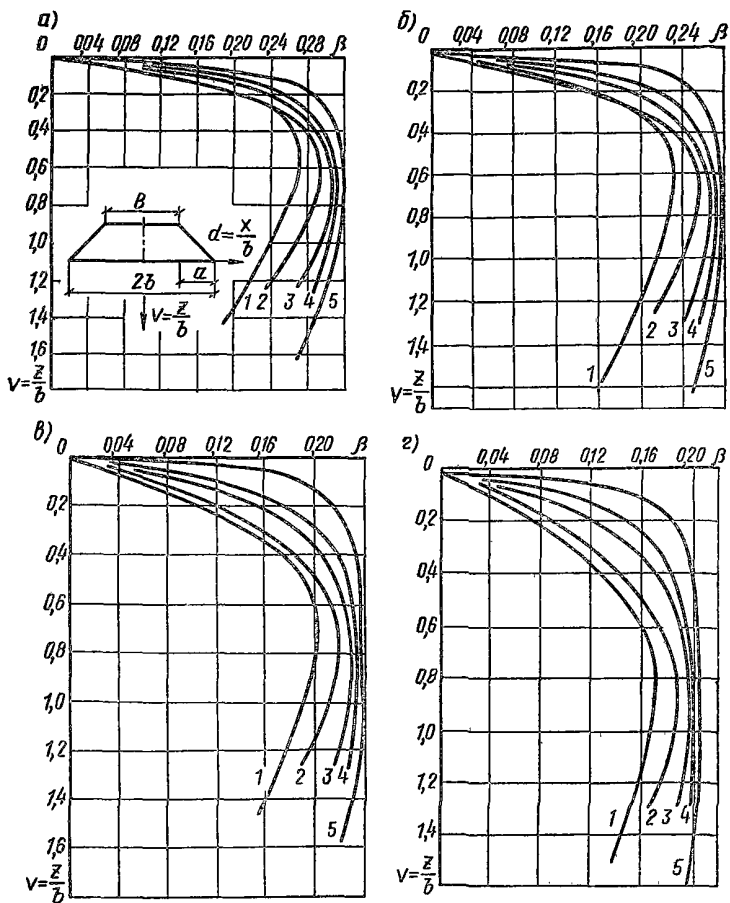
Рис. 7. График функций \beta при:
