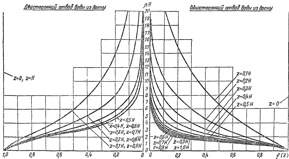
Рис. 2. График зависимости \beta H от f(z) для различных значений z
