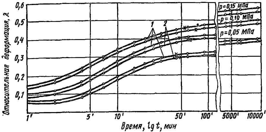
Рис. 9. Кривые консолидации
