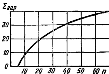
Рис. 5. График для определения гарантированной частоты \Sigma_{гар} в зависимости от числа определений n показателей физико-механических свойств грунтов
