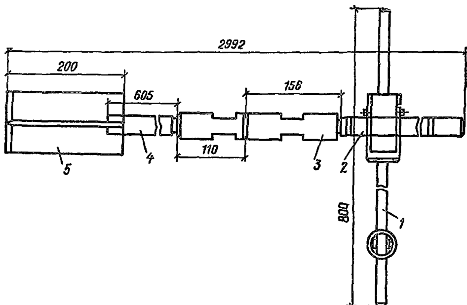
Рис. 4. Лопастной прибор БЕЛДОРНИИ для определения сопротивления сдвигу торфяных грунтов
