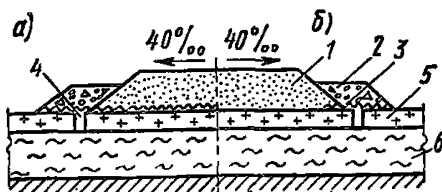
Рис. 22. Конструкция насыпи с прорезями, перекрытыми прослойкой из геотекстильного материала, проложенной
