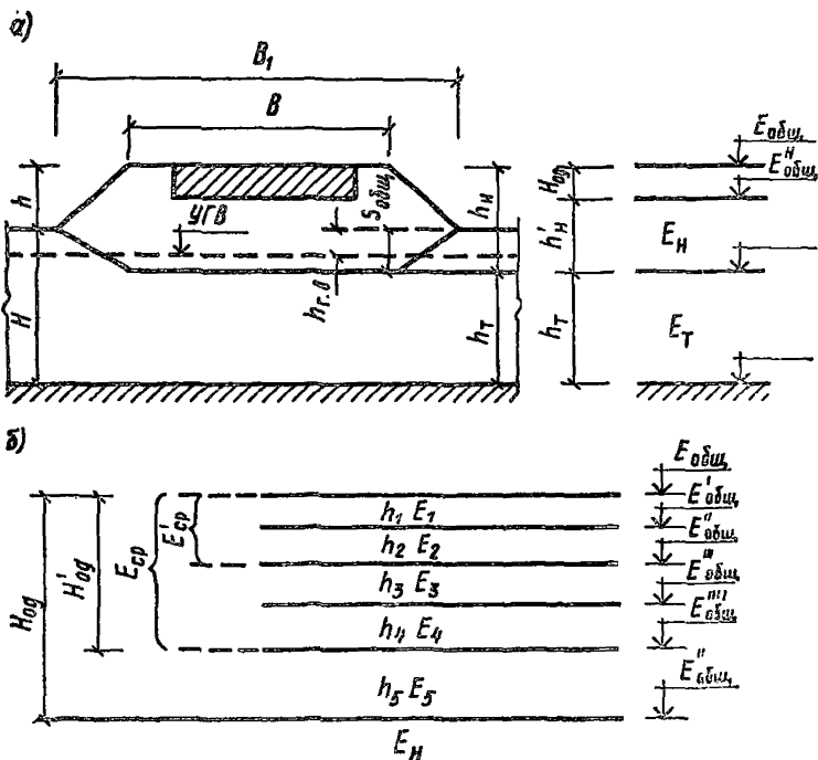
Рис. 1. Расчетная схема
