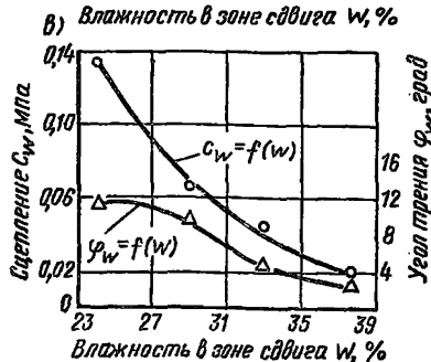
Рис. 13. Пример обработки сдвиговых испытаний
