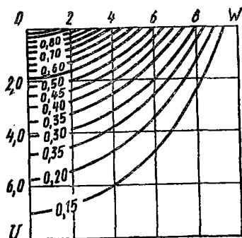
Рис. 13. Графики значений \alpha_2 = \sigma_2/\rho_0 при 2a/B=10
