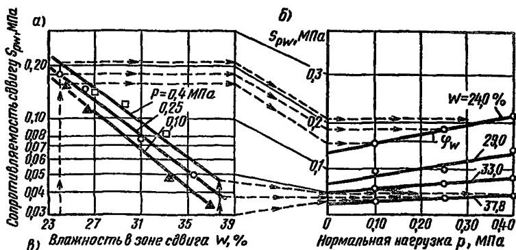
Рис. 13. Пример обработки сдвиговых испытаний
