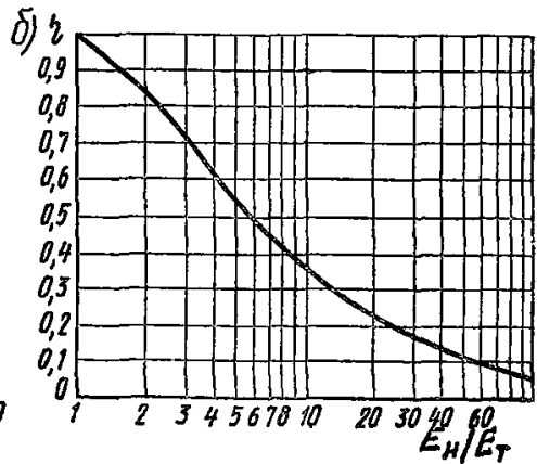
Рис. 4. Графики для определения коэффициентов k и \eta
