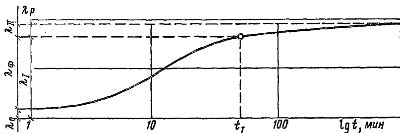
Рис. 10. Общий вид кривой консолидации
