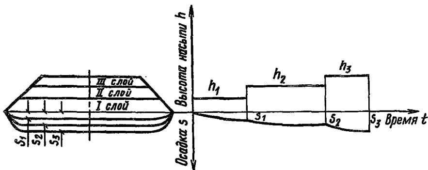
Рис. 19. Схема возведения насыпи методом постепенного нагружения (предварительной консолидации)
