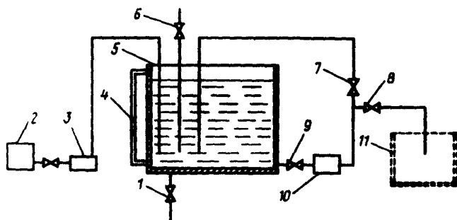
Рис.2. Схема приготовления раствора катализатора: 1,6,7,8,9-вентили; 2-емкость с катализатором; 3-ручной насос; 4- водомерная трубка; 5-бак для раствора катализатора; 10-электронасос; 11-привозная емкость (для раствора катализатора)
