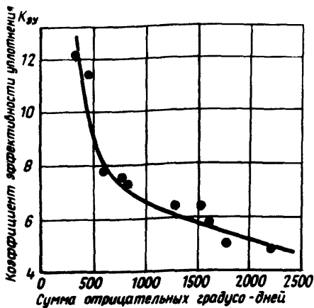
Рис.8. Зависимость коэффициента эффективности утепления грунта K_{\Sigma} БТП от суммы отрицательных градусо-дней
