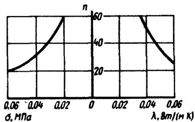
Рис.2. Зависимость прочности \sigma и теплопроводности \lambda пенопласта от его кратности n
