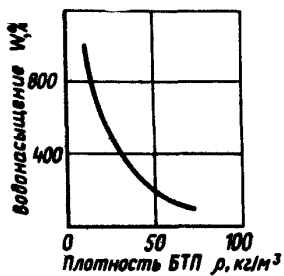
Рис.3. Влияние плотности \rho БТП на его водонасыщение W
