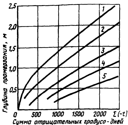
Рис.9. Зависимость глубины промерзания грунта от суммы отрицательных градусо-дней и толщины снегового покрова или ледяного покрова 1-0 м; 2-0,2 м; 3-0,2-0,4 м; 4-0,4-0,6 м; 5- выше 0,6 м
