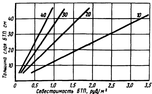
Рис.11. Зависимость себестоимости утепления от толщины слоя БТП и кратности пены (цифры на кривых)
