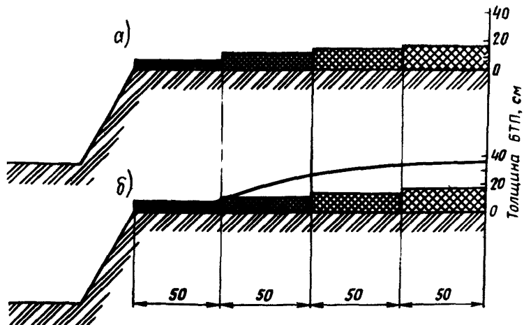
Рис.10. Схема проведения теплоизоляции карьера в Московской обл. ( H_{пр}=140 см): а-утепление БТП и снегом (пенольдом) при их средней толщине 20 см; б-утепление только БТП
