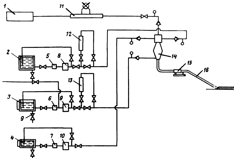
Рис.2. Принципиальная схема установки УПС-100 конструкции Союздорнии и Ленинградского филиала Союздорнии: 1-компрессор; 2-бак для эмульсии смолы с пенообразователем; 3-бак для кислоты; 4-бак для воды; 5,6,7-фильтры; 8,9,10-насосы; 11-расходомер для воздуха; 12,13-расходомеры для растворов; 14-пенногенератор; 15-распределительное устройство; 16-пенопровод
