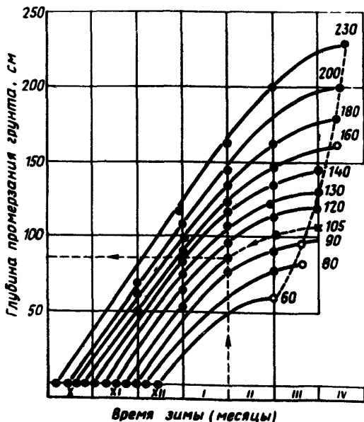
Рис.7. Ход изменения глубины промерзания грунта во времени. Цифры на кривых – нормативная глубина промерзания в конце зимы, см
