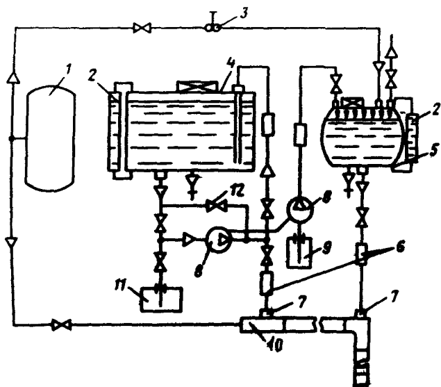
Рис.4. Принципиальная схема установки ПГУ конструкции СибНИИГиМа: 1-компрессор; 2-указатели уровня; 3-редуктор; 4-бак для эмульсии смолы с пенообразователем; 5-бак для кислоты; 6-расходомеры; 7-обратные клапаны; 8-насосы; 9-тара с кислотой; 10-пеногенератор; 11-тара со смолы; 12-перепускной клапан
