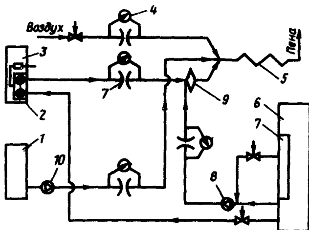
Рис.3. Принципиальная схема машины ПГМ-120; 1-бак для кислоты; 2-насос для подачи смолы; 3-бак для смолы; 4-дифманометр; 5-пеногенератор; 6-бак для воды; 7-бак для пенообразователя; 8-насос для подачи воды; 9-смеситель; 10-насос для подачи кислоты
