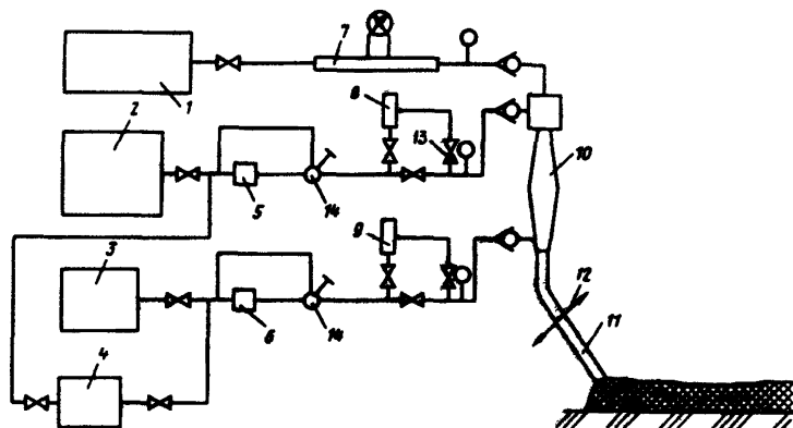
Рис.5. Принципиальная схема пеногенераторной установки УПС-80 конструкции Союздорнии и Ленинградского филиала Союздорнии: 1-компрессор; 2-бак для эмульсии смолы; 3-бак для кислоты; 4-бак для воды; 5,6-насосы; 7-расходомер воздуха; 8,9-расходомеры растворов; 10-пеногенератор; 11-пенопровод; 12-распределительное устройство; 13-вентили; 14-регулятор расхода
