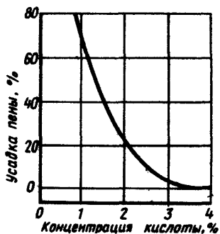
Рис.1. Влияние концентрации кислоты на усадку пены
