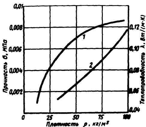
Рис.4. Зависимость прочности \sigma (1) и теплопроводности \lambda (2) пенольда от его плотности \rho
