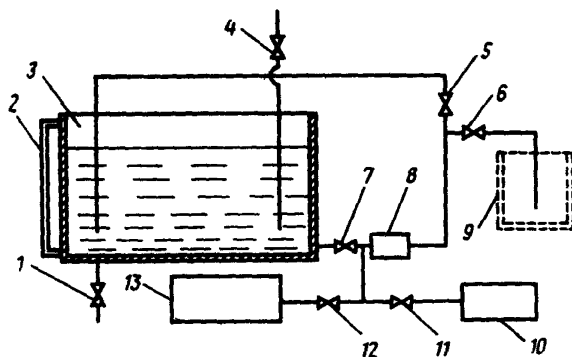
Рис.1. Схема приготовления раствора смолы и пенообразователя: 1,4,5,6,7,11,12- вентили; 2- водомерная трубка; 3-бак для раствора; 8-электронасос; 9-привозная емкость для раствора; 10-емкость с пенообразователем; 13-емкость со смолой
