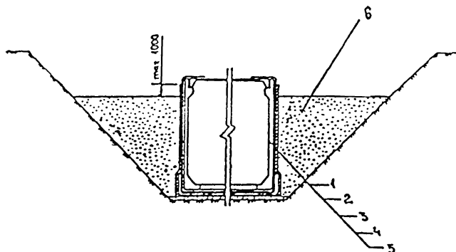
Рис. 21. Защита гидроизоляции стен:
