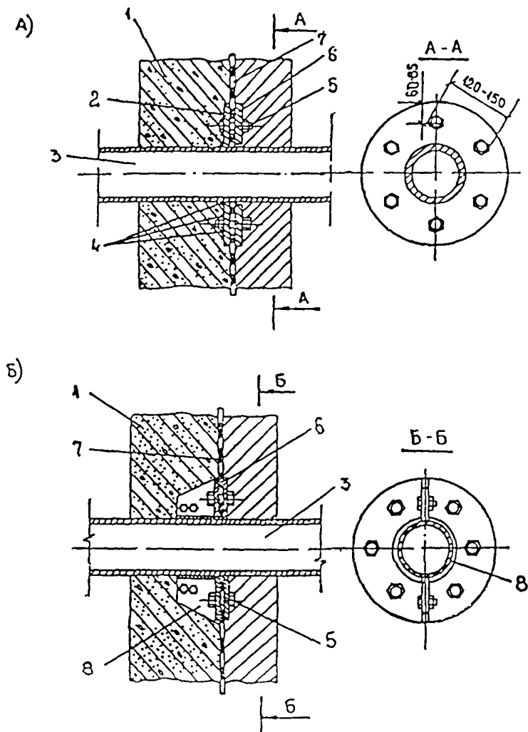
Рис. 19. Сопряжение гидроизоляции с трубопроводом: а — стальным; б — чугунным; 1 — бетон; 2 — фланец приварной; 3 — труба; 4 — водонепроницаемый сварной шов; 5 — болт; 6 — фланец накладной; 7 — гидроизоляция; 8 — хомут
