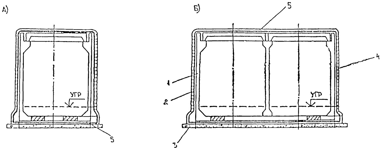
Рис. 1. Общий вид тоннеля с гидроизоляцией:
