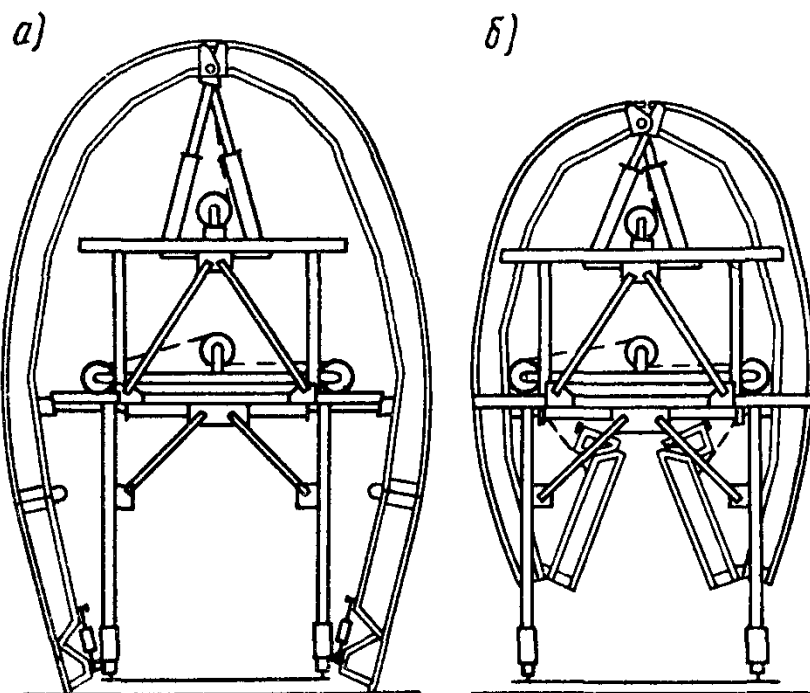
Рис. 2. Опалубочная тележка: a —установленная опалубочная секция, б —перемещаемая опалубочная секция
