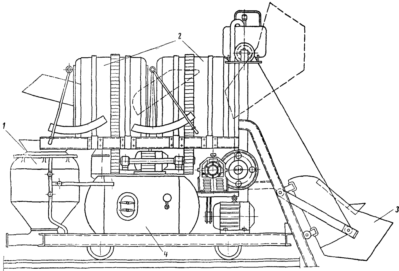
Рис. 2. Бетонукладочный агрегат с пневмобетонагнетателем: 1—пневмобетонагнетатель; 2—бетоносмесительное устройство; 3—скип; 4—ресивер
