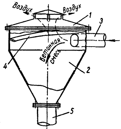
Рис. 9. Схема гасителя: 1—крышка; 2—корпус; 3—входной патрубок; 4—отбойный лист; 5—гиб- кий шланг
