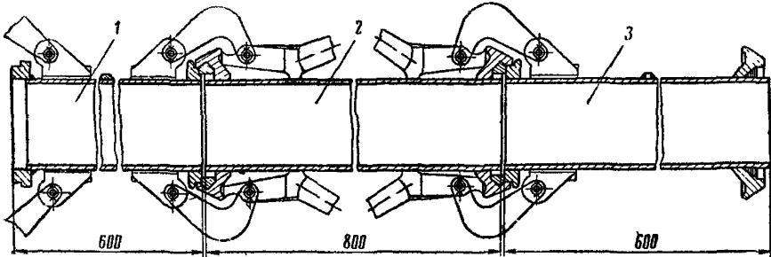
Рис. 7. Быстроразъемная секция: 1—левое звено; 2—среднее звено; 3—правое звено
