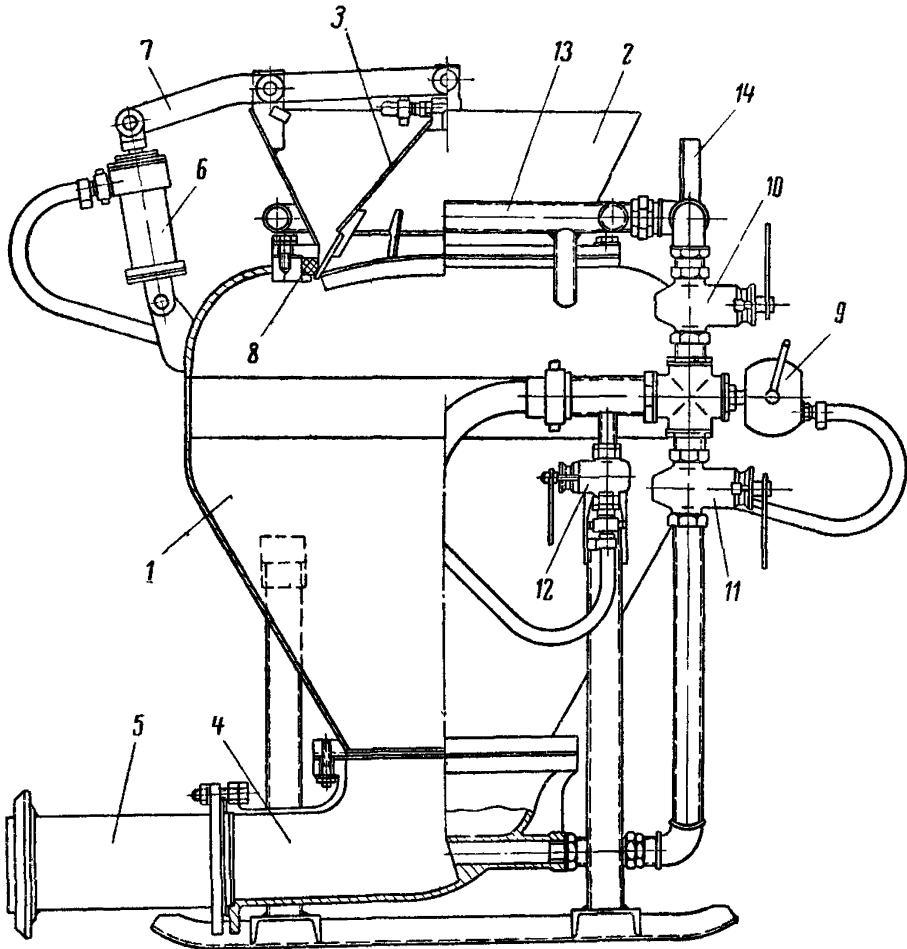
Рис. 1. Схема пневмобетонагнетателя:
