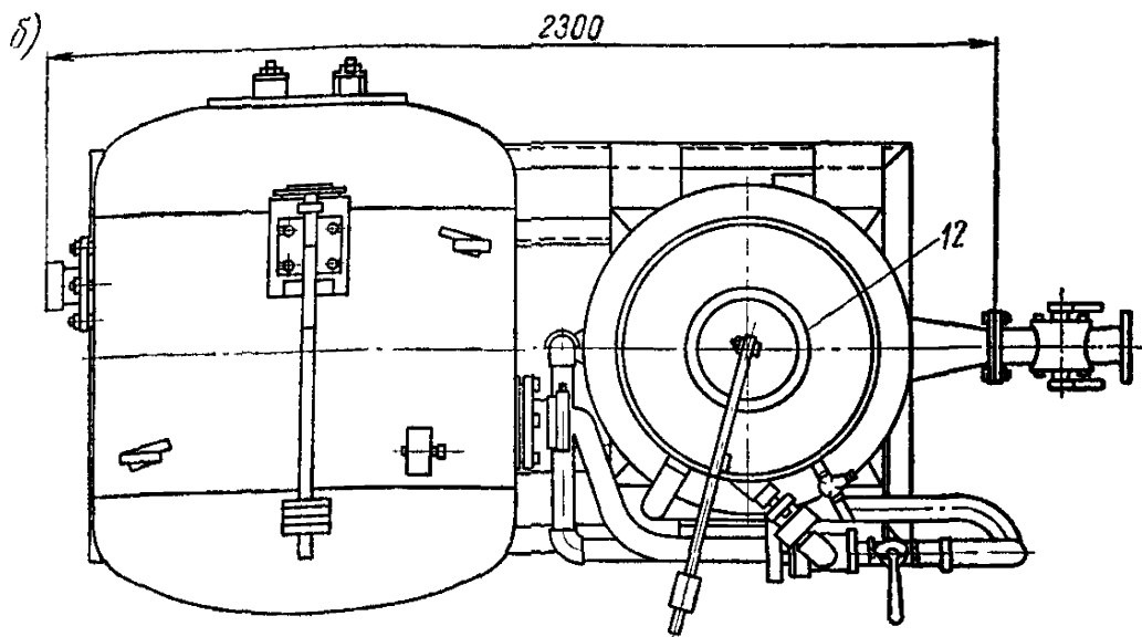
Рис. 4. Общий вид пневматической установки С-862:
