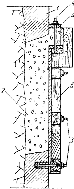
Схема опалубки для заполнения бетоном дефектных мест тоннельной обделки
