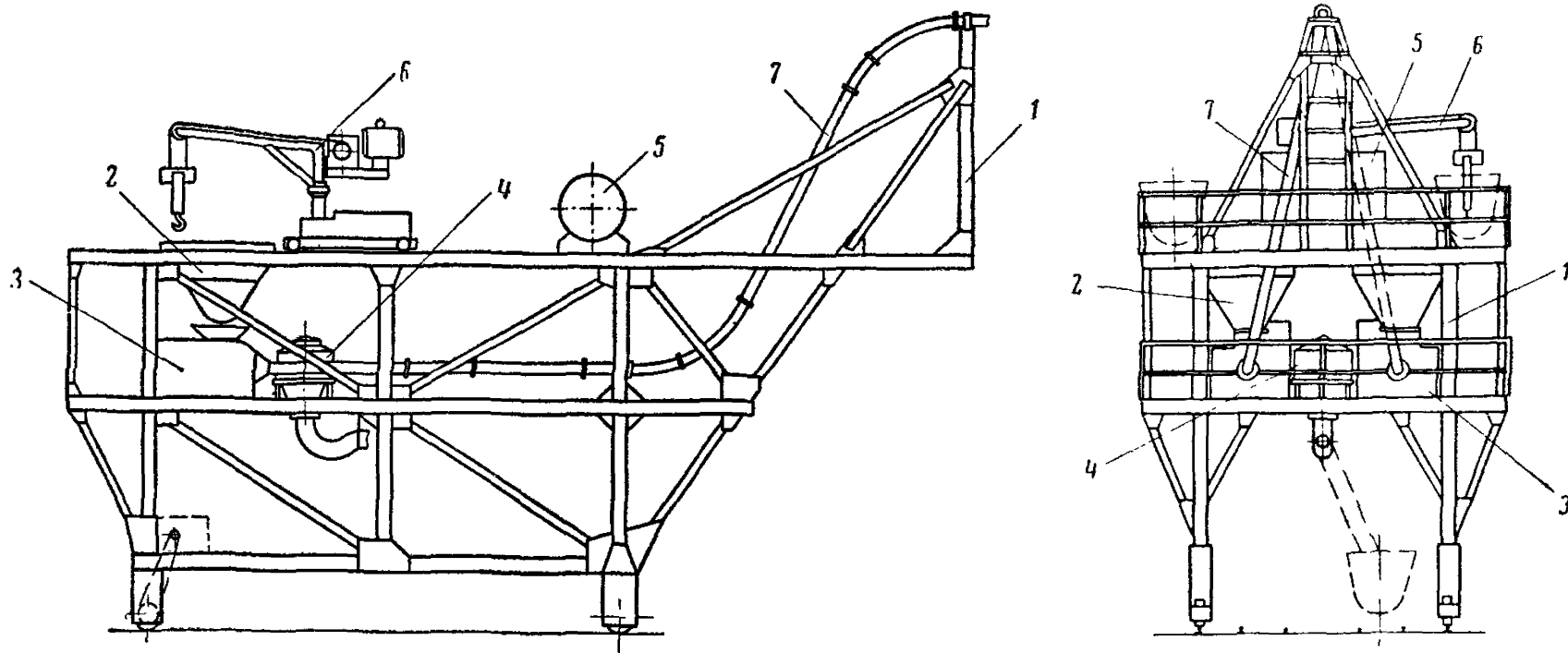
Рис. 5. Бетноукладочная установка:
