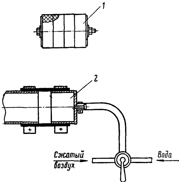
Рис. 8. Вспомогательные устройства: 1—пыж; 2—продувочный патрубок
