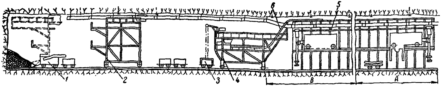
Рис. 11. Технологическая схема возведения обделки с использованием сборно-разборной опалубки, установленной за буровой рамой: 1—погрузочная машина; 2—буровая рама; 3—бетоновозка; 4—бетоноукладочная установка; 5—сборно-разборная опалубка; 6—бетоновод
