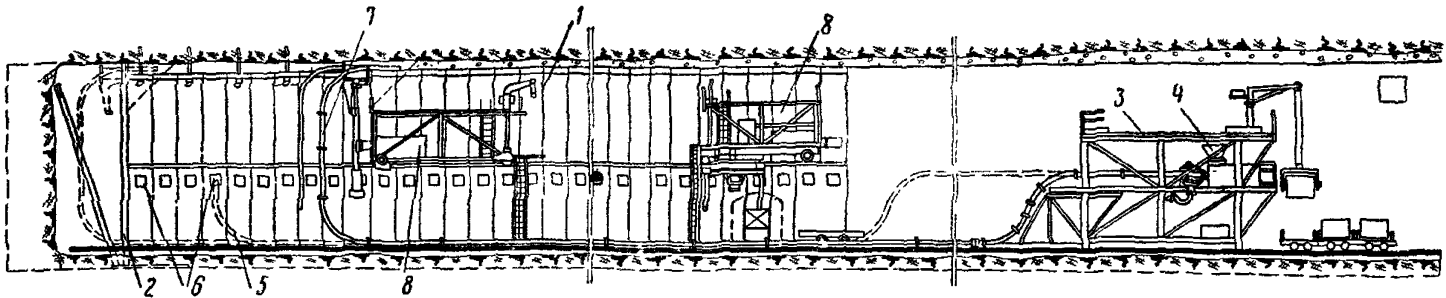
Рис. 12. Технологическая схема возведения обделки с применением сборно-разборной опалубки у забоя: 1—опалубка; 2—торцовая рама; 3—бетоноукладочная установка, 4—бетоноукладочная машина; 5 и 7—бетоноводы; 6—люки в опалубке; 8—перестановщики
