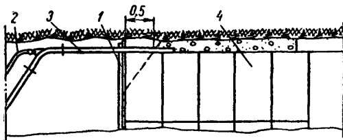
Рис. 17. Укладка бетонной смеси в свод обделки: 1—торцевая рама; 2—устройство для подачи сжатого воздуха; 3—бетоновод; 4—опалубка
