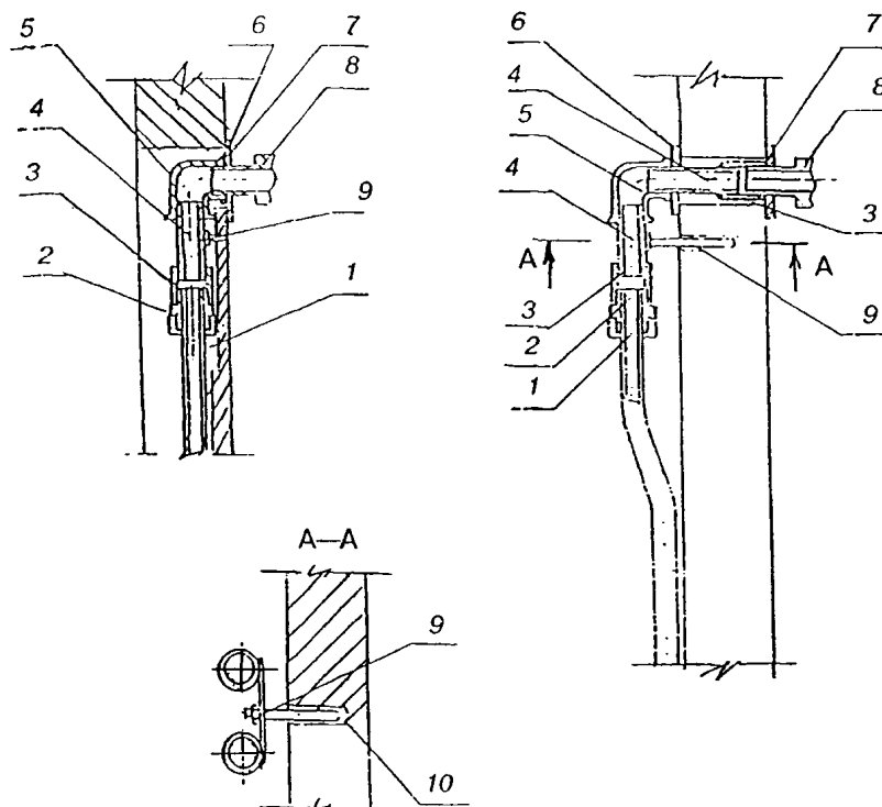
1 — подводка из металлополимерной трубы; 2 — соединительная деталь; 3 — муфта стандартная; 4 — патрубок из стальной трубы; 5 — угольник стандартный; 6 — шайба упорная; 7 — шайба декоративная; 8 — арматура водоразборная; 9 — крепление; 10 — дюбель
