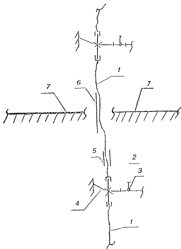
1 — междуэтажная вставка из МПТ 2025; 2 — латунный тройник; 3 — вентиль; 4 — неподвижное крепление; 5 — подвижное крепление; 6 — гильза; 7 — междуэтажное перекрытие
