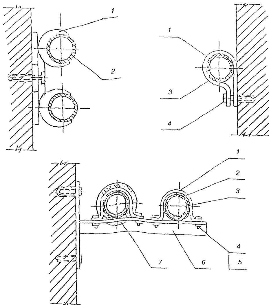
1 — хомут металлический; 2 — труба металлополимерная; 3 — прокладка резиновая; 4 — болт; 5 — гайка; 6 — кронштейн; 7 — теплоизоляция
