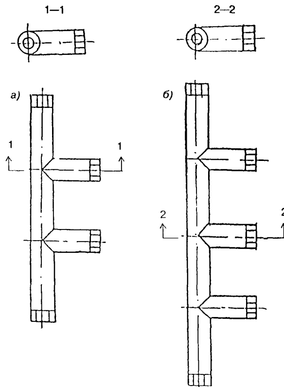
а — с односторонним прямым расположением 2 отводящих штуцеров; б — с односторонним прямым расположением 3 отводящих штуцеров
