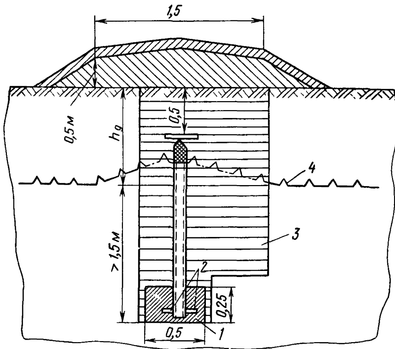
Рис. 2. Схема устройства грунтового репера для применения на участках с несליвающейся мерзлотой:
