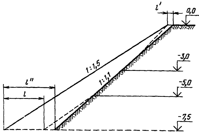
Рис 2 Расчетная схема проектирования обсыпки (к примеру)
