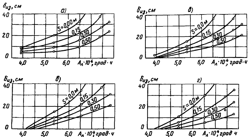
Рис. 4. Зависимость толщины слоя пенопласта \delta_{из} от суммы градусочасов приведенных температур воздуха за теплый период A_{л} и допустимой глубины оттаивания грунта под теплоизоляцией s при укладке пенопласта:
