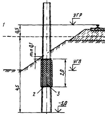
Рис 12 Схема установки опоры контактной сети с противоучин- ной обмоткой 1—уровень условного обреза фунда- мента 2—хомут (скрутка) 3—обмотка (3 слоя полиэтилена и 3 слоя несмер- зающей смазки например ЦИАТИМ 201)
