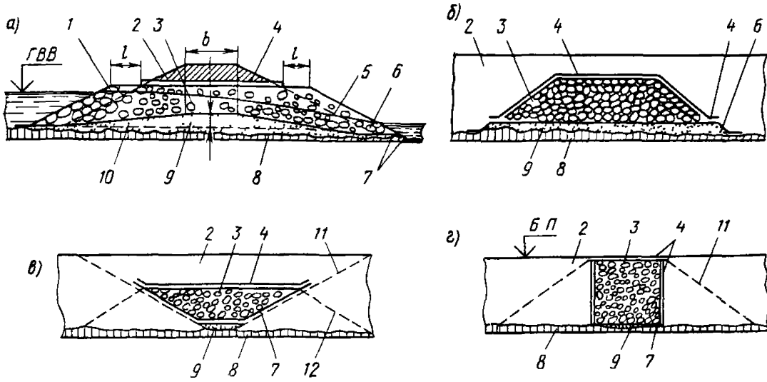
Рис. 2. Схема устройства ФН на слабом основании, в том числе на марях: а —продольный разрез; б —поперечный разрез ФН, сооружаемой до возведения прилегающих участков земляного полотна; в —то же после возведения насыпи; г —то же, сооружаемой в условиях эксплуатации дороги; 1 —входной оголовок ФЧ, выступающий за плоскость откосов дорожной насыпи в виде берм шириной l ; 2 —дорожная насыпь; 3 —ФЧ сооружения, 4 —изоляция верха и боков ФЧ (синтетический нетканый материал типа дорнит); 5 —кривая депрессии водного потока в пределах ФЧ сооружения; 6 —выходной оголовок ФЧ; 7 —изоляция верха и боков подушки и откосов подходов насыпи, 8 —растительно-моховой покров; 9 —подушка из песка или галечно-гравийного грунта высотой над верхом кочек под основной площадкой h , отсыпаемая на поверхность растительно-мохового покрова; 10 —условный уровень верха кочек; 11 —откосы подходов насыпи до возведения ФЧ сооружения; 12 —откосы оголовков ФЧ сооружения; Б п —отметка бровки полотна
