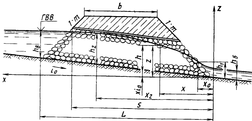
Схема к гидравлическому расчету безнапорной ФН
