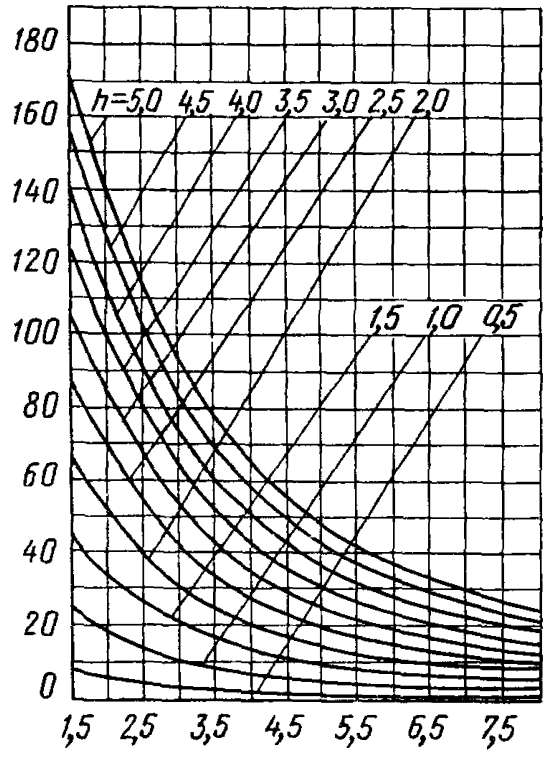
Рис 1 Кривые изменения значений функции K_q для вагонов: а—четырехосных; б—шестиосных; в—восьмиосных
