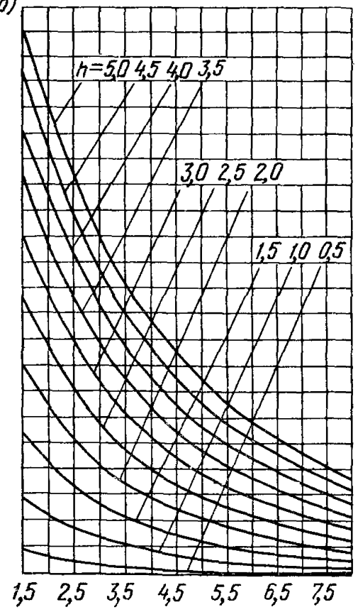
Рис 1 Кривые изменения значений функции K_q для вагонов: а—четырехосных; б—шестиосных; в—восьмиосных
