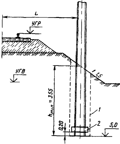
Рис 11 Схема размещения и за- крепления фундаментов опор на участках с неблагоприятными мерзотно грунтовыми условиями (см табл 6) 1—контур котлована 2—анкерная плита
