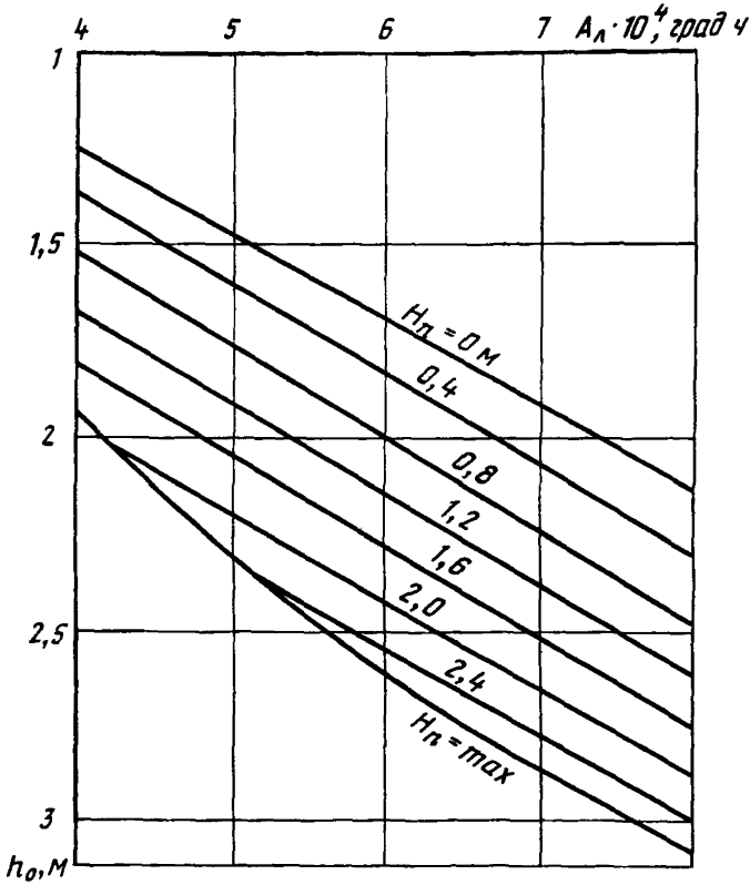
Рис 3. Номограмма для определения глубины сезонного оттаивания грунта в зависимости от градусо-часов температуры воздуха за теплый период A_d и величины песчаного слоя на поверхности H_n
