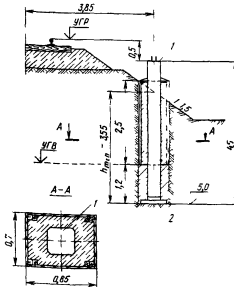
Рис 12 Схема установки опоры контактной сети с противоучин- ной обмоткой 1—уровень условного обреза фунда- мента 2—хомут (скрутка) 3—обмотка (3 слоя полиэтилена и 3 слоя несмер- зающей смазки например ЦИАТИМ 201)
