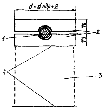
Рис 2 Шарнирное устройство:
