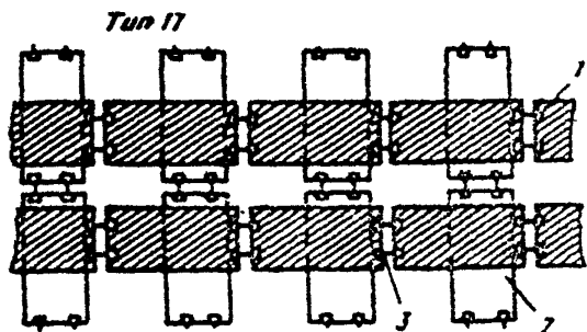
Рис.10. Усиление ледовой переправы клефанерным дорожным покрытием: 1—плита основного пути; 2—поперечно уложенные плиты; 3—монтажные стыки
