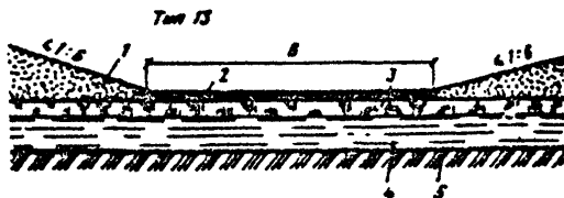
Рис.7. Поперечный профиль автозимника на ледяном покрове рек и озер (морей): 1-снежный покров; 2-уплотненный слой снега толщиной 3-5 см на плотне; 3-ледяной покров; 4-вода; 5-дно водоема
