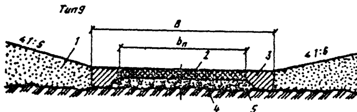
Рис. 4. Поперечный профиль автозимника на марях и бугристых вечномерзлых торфяниках: 1—снежный покров; 2—уплотненный или оледеневший снег на проезжей части; 3—уплотненный снег на обочинах; 4—выравнивающий слой из гравия или песка; 5—спланированное мерзлое основание
