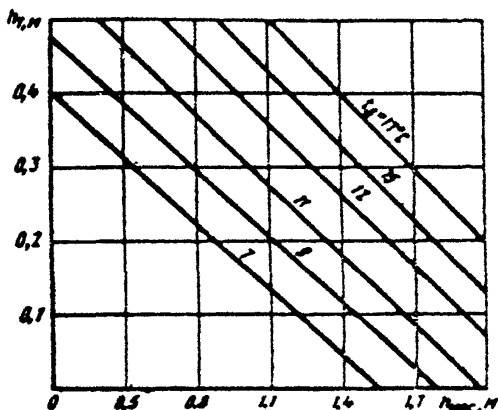
Рис.18. Определение высоты насыпи h_{нас} из песчаных грунтов или толщины слоя теплоизоляции h_t из торфа
