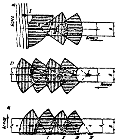
Рис.19. Намораживание ле - довых переправ методом дождевания: а-с берега ; б-при движении агрегата по оси переправы; в-то же, вдоль переправы; • - кон - трольные вехи; ▨ - стоянки агрегата; ▩ - секторы дож - девания; ▨▨ - перекрывае мые зоны; 1-1У - последователь - ные стоянки (позиции) агре - гата
