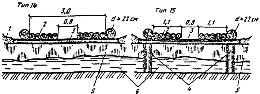
Рис. 8. Усиление ледовых переправ деревянным настилом: 1—снежный покров; 2—колесопроводы, d > 22 см; 3—поперечины, d > 18 см; 4—стойки, d > 20 см; 5—естественный ледяной покров; 6—вода
