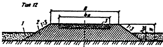
Рис.6. Поперечный профиль автозимника в насыпи из снега: 1-снежный покров толщиной h_{см} ; 2-насыпь из уплотненного снега; 3-оледененный слой снега на проезжей части; H -высота насыпи
