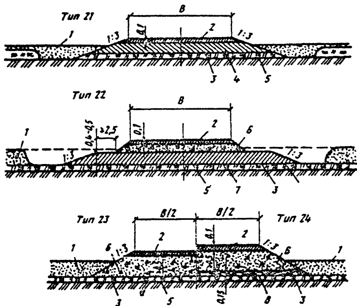
Рис. 14. Поперечные профили автозимников с продленными сроками эксплуатации: 1-снежный покров; 2-уплотненный слой снега на полотне дороги; 3-естественный мохорастительный покров; 4-теплоизолирующее полотно из снега со мхом; 5-мерзлое грунтовое основание; 6-земляное полотно; 7-полотно из уплотненного снега; 8-слой теплоизоляции или хворостяная выстилка
