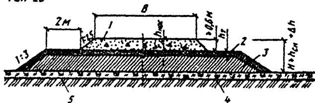
Рис.15. Поперечный профиль автозимника для круглогодичной эксплуатации: 1—земляное полотно из минерального грунта; 2—слой теплоизоляции из торфа, мха, опилок и т.п.; 3—снежно-ледяное ядро; 4—естественный мохорастительный покров; 5—мерзлое грунтовое основание
