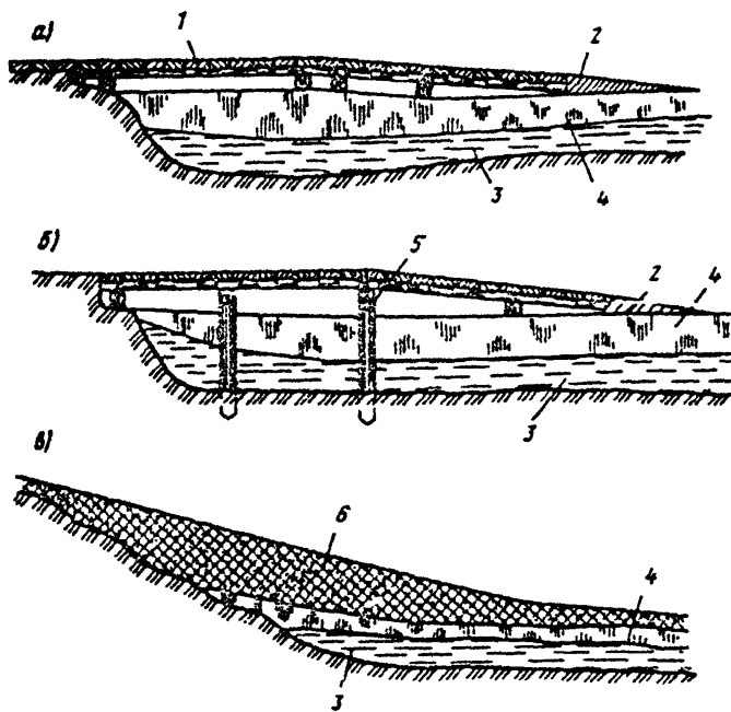
Рис.13. Конструкции сопряжения берега и ледяного покрова на переправах: а-простейший съезд с берега на лед; б-свайный съезд; в-съезд, намороженный способом дождевания; 1-настил; 2-лед с замороженным хвостом; 3-вода; 4-естественный ледяной покров; 5-стойки; 6-намороженный слой льда
