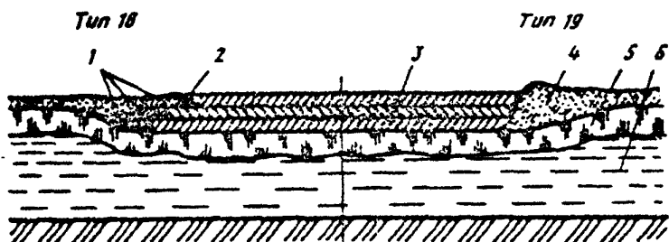
Рис.11. Усиление ледяного покрова методом послойного намораживания льда: 1—пригравированный снег; 2—жерди; 3—намораживаемые слои; 4—вал из снега; 5—естественный ледяной покров; 6—вода
