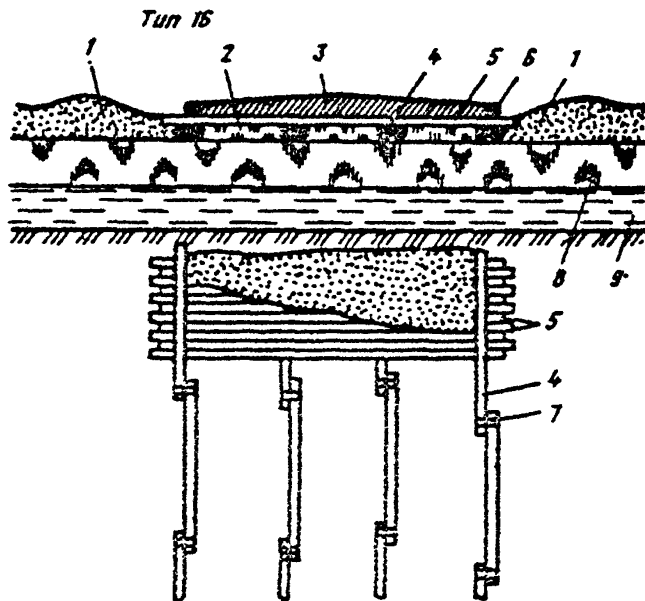
Рис. 9. Конструкция "плавающей" дереволедяной переправы: 1—валик из снега; 2—намороженный слой льда; 3—снежно-ледяное полотно; 4—продольные лежни, a > 20 см; 5—сланевый настил из тонкомерной древесины; 6—колесоотбой, d > 22 см; 7—проволочная скрутка \Phi=8 мм; 8—естественный ледяной покров; 8—вода
