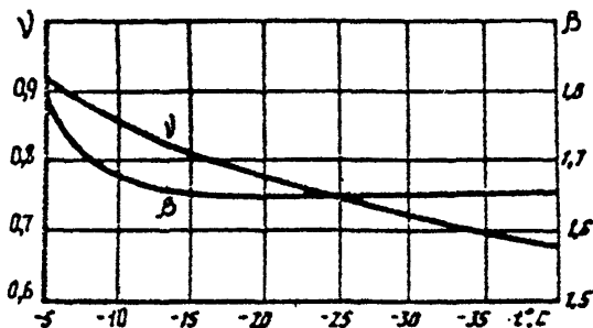
Рис.24. Графики для определения коэффициентов \gamma и \beta
