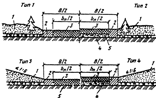
Рис.1. Поперечные профили автозимников на прочных грунтовых основаниях: 1—снежный покров; 2—уплотненный снег на обочинах; 3—уплотненный или оледеневший снег на проезжей части; 4—выравнивающий слой из гравия, щебня или песка; 5—спланированное основание
