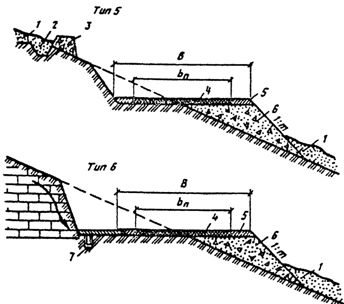
Рис.2. Поперечные профили автозимников на косо- горах: 1—снежный покров; 2—нагорная канава; 3—нагорный валик; 4—уплотненный или оледененный снег на проезжей части; 5—уплотненный снег на обочинах; 6—грунтовая насыпь на косогоре; 7—утепленный лоток для отвода грунтовых вод ; — — направление движения грунтового потока
