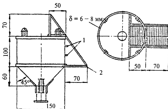
Рис. 30. Конструкция приемной воронки объемом 2 м 3 с площадками:
