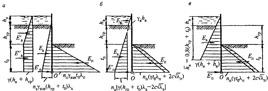
Рис. 17. Схема, используемая в расчетах шпунтовых ограждений, не имеющих распорных креплений, и эпюры давлений:
