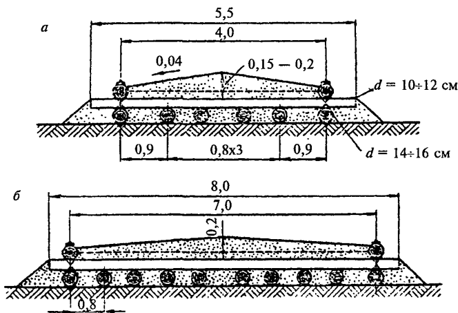
Рис. 7. Типы лежнево-сланевой дороги:
