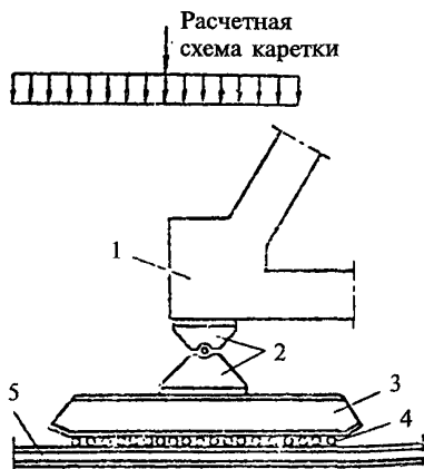
Рис. 54. Опираие узла пролетного строения на накаточные пути при продольной надвигке на плаву:
