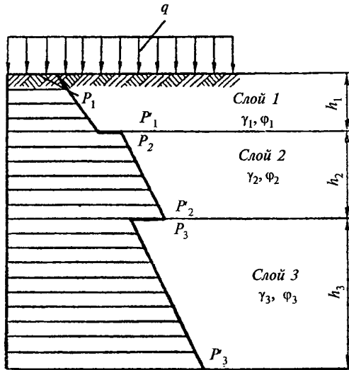
Рис. 8. К определению активного давления грунта из нескольких слоев песка или суглинка на стенку ограждения
