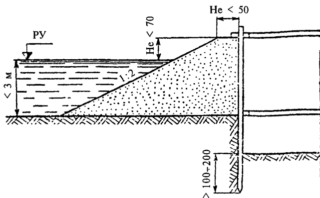
Рис. 10. Шпунтовая однорядная перемычка с односторонней отсыпкой грунта
