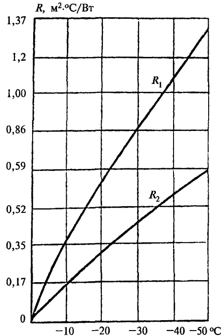
Рис. 37. Кривые зависимости оптимального термического сопротивления боковых поверхностей опоры R ( \text{м}^2\cdot\text{°C}/\text{Вт} ) от расчетной температуры наружного воздуха, \text{°C} ( R_1 — для торцовых поверхностей и боковых частей поверхности, прилегающих на 2 м к углам опоры; R_2 — для остальных частей боковых поверхностей)
