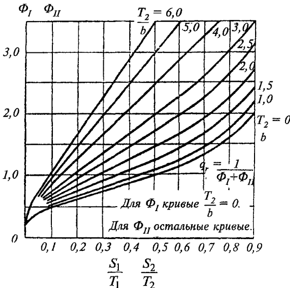
Рис. 2. График для определения q_r = f\left(\frac{S_1}{T_1}; \frac{S_2}{T_2}\right) в случае близкого расположения водоупорного слоя ( \Phi_I определяется в функции \frac{S_1}{T_1} ; \Phi_{II} — в функции \frac{S_2}{T_2} )
