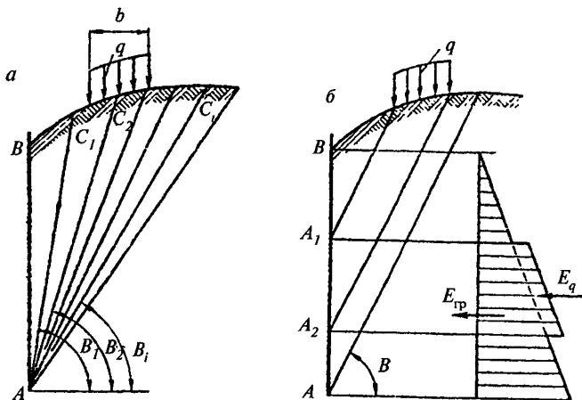
Рис. 7. К определению активного давления песка или супеси на стенку ограждений при произвольном очертании поверхности грунта и расположении на ней нагрузки
