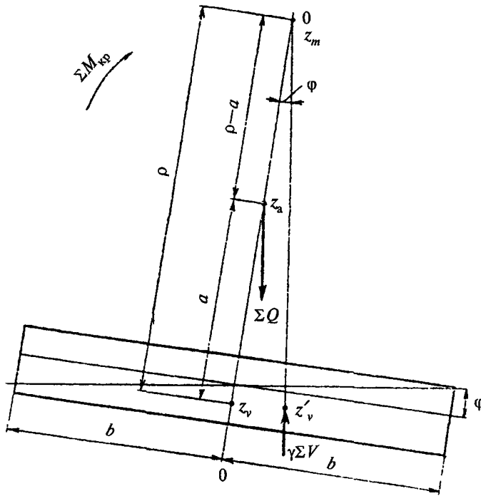
Рис. 56. Схема определения остойчивости плавучей опоры
