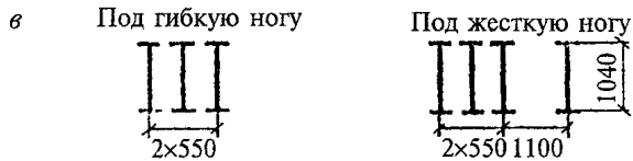
Рис. 1. Примерные монтажные схемы пакетных пролетных строений:
