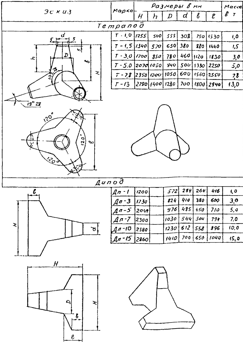
Рисунок 7.9 - Технические характеристики фасонных массивов
