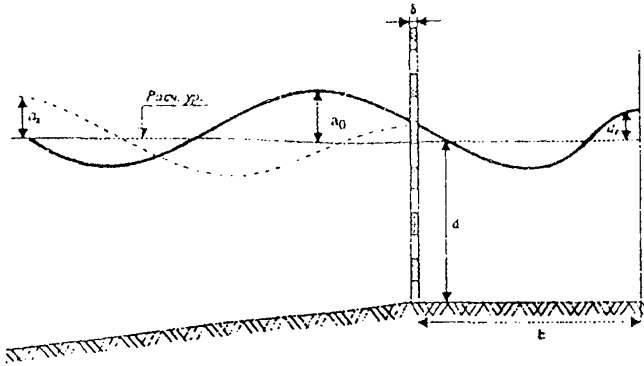
Рисунок 6.3 - Взаимодействие волн с пропускаемым сооружением: d - глубина воды у стенки; \delta - толщина пропускаемой стенки; b - ширина волновой камеры; a_0 - амплитуда подходящих волн; a_1 - амплитуда прошедших волн; a_2 - амплитуда отраженных волн
