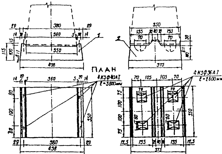
Рисунок 7.23 - Варианты конструкций подставок: 1 - старая; 2 - новая
