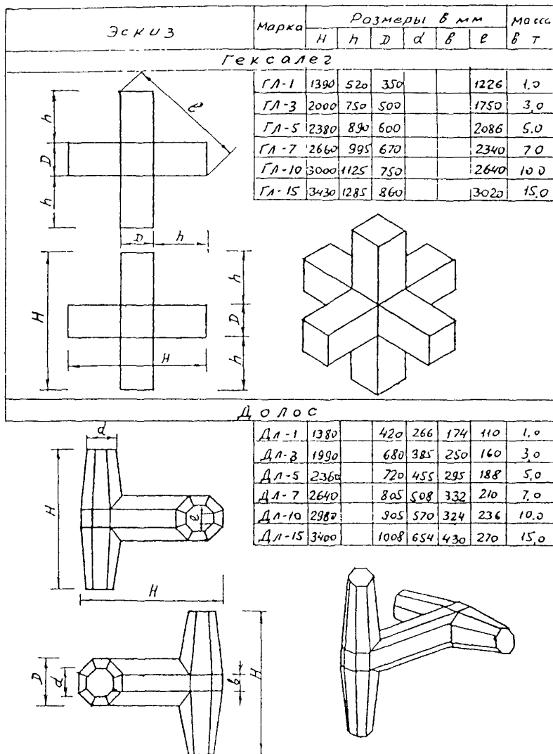
Рисунок 7.10 - Технические характеристики фасонных массивов
