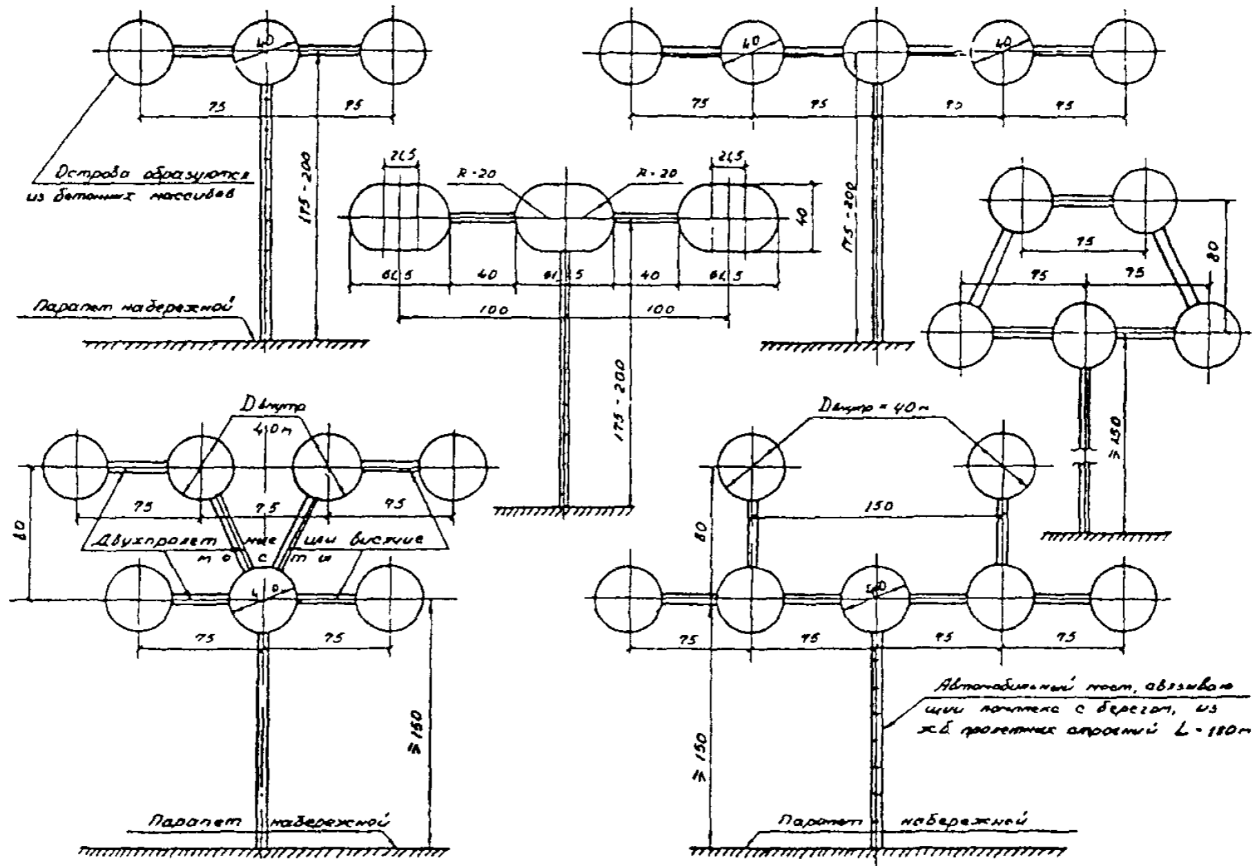
Рисунок 8.3 - Схемы вариантов островных комплексов в плане
