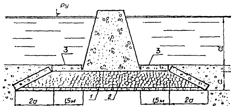
Рисунок 7.22 - Каменная постель под гравитационной бунной: 1 - подготовка из щебня толщиной слоя 0,3-0,5 м; 2 - камень со средним размером 35-50 см; 3 - берменная плита
