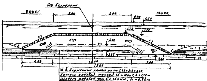
Рисунок 7.27 - Поперечное сечение волнолома распластанной конструкции
