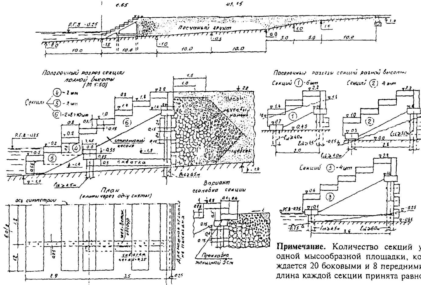
Рисунок 8.2 - Поперечный разрез по оси мысообразной площадки (М 1:200)
