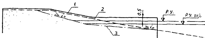
Рисунок 7.15 - Схема профиля буны на берегу с песчаными наносами: 1 - гребень буны; 2 - профиль проектного пляжа с верхней стороны буны; 3 - то же с нижней стороны буны
