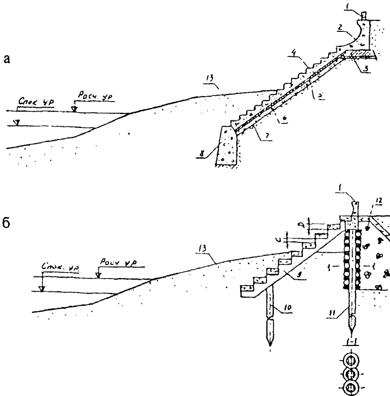
Рисунок 7.8 - Схемы откосно-ступенчатого укрепления:
