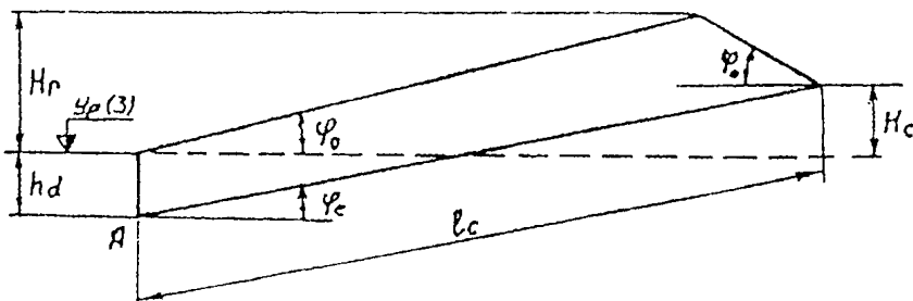
Рисунок 6.5 - Расчетная схема надвига льда на откос сооружения
