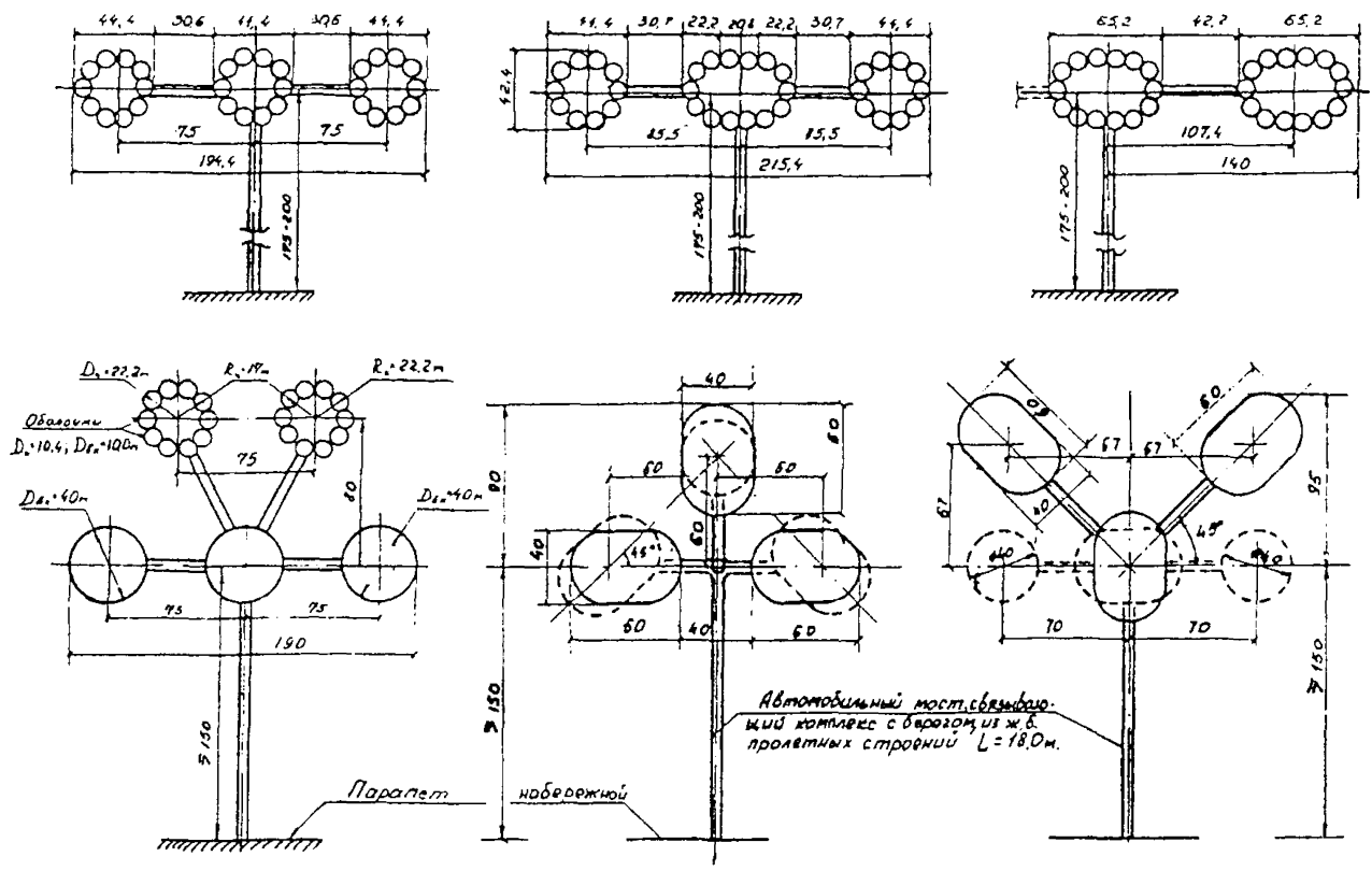
Рисунок 8.4 - Схемы вариантов островных комплексов в плане
