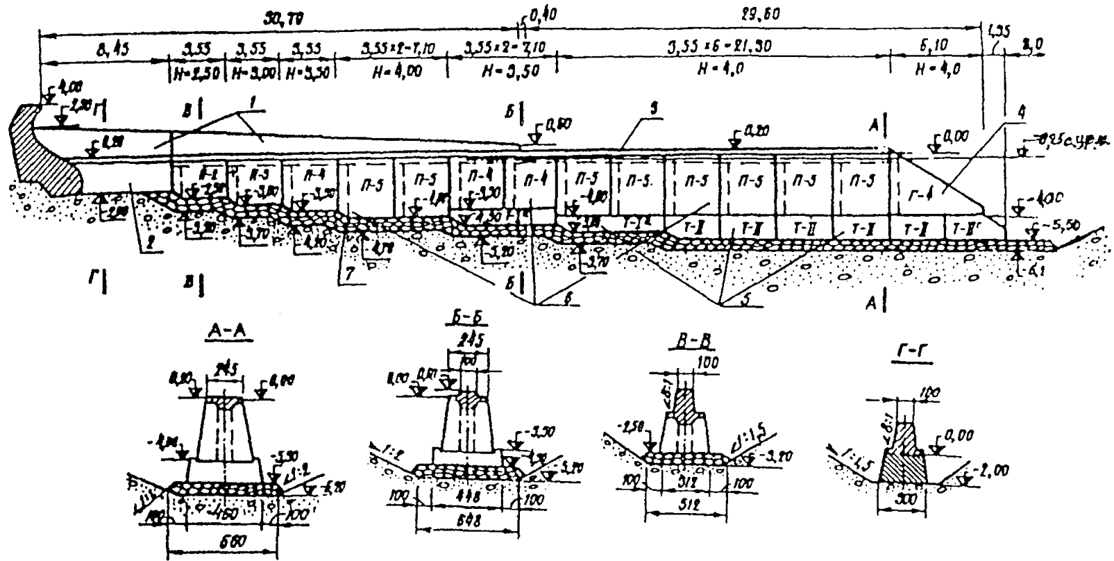
Рисунок 7.20 - Конструкция буны на размываемом основании:
