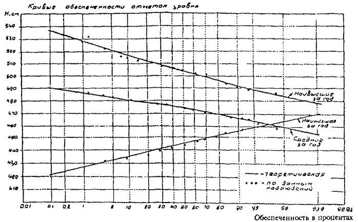
Рисунок 5.1 - Кривые обеспеченности отметок уровня моря
