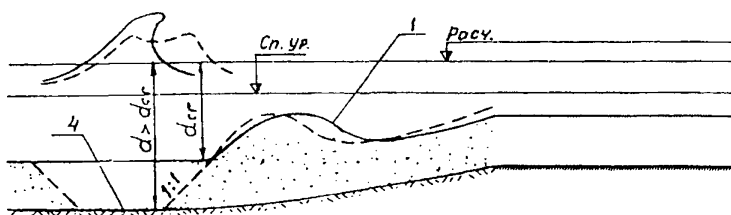
Рисунок 8.5 - Способ берегозащиты свободным пляжем с устройством перед ним подводной траншеи: 1 - свободный пляж; 2 - свободный пляж с траншеей; 3 - клиф; 4 - траншея
