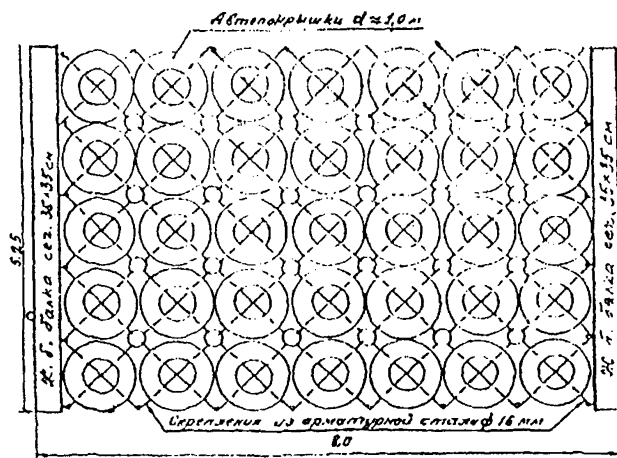
Рисунок 7.28 - Конструкция защитного «ковра» из автопокрышек
