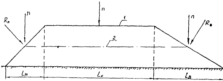
Рисунок 7.2 - Плановое положение искусственного свободного песчаного пляжа:
