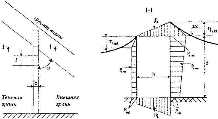
Рисунок 6.1 - Эпюры волнового давления на буну
