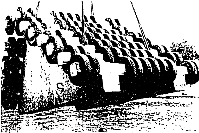
Рисунок 7.35 - Блок волнолома проникаемой конструкции с покрывками массой 90 т
