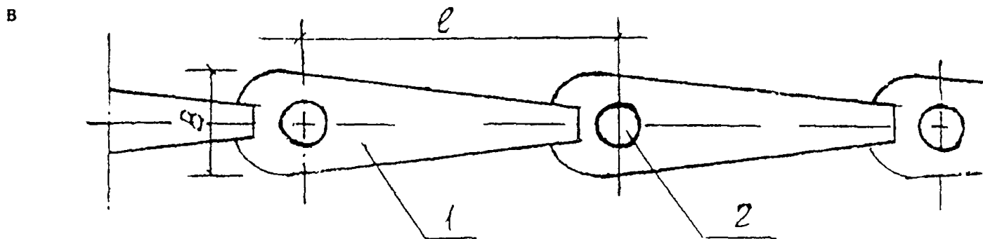
Рисунок 7.19 - Продолжение: б) фрагмент тонкостенной буны в плане: 1 - промежуточный блок; 2 - ж.б. плита-экран; 3 - колонна-оболочка. в) фрагмент буны из «каплевидных» массивов в плане: 1 - «каплевидный» массив; 2 - колонна-оболочка
