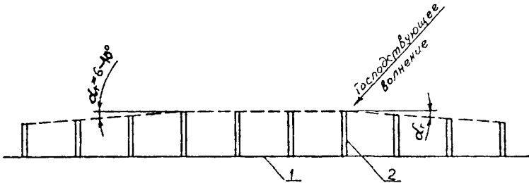
Рисунок 7.16 - Схема уменьшения длины буны на концевых участках системы в условиях песчаных пляжей: 1 - берег; 2 - бунна; \alpha_g - угол отклонения линии головных частей бун
