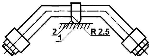
Устройство для вдавливания шарика: 1 - образец; 2 - сферическая часть (шарик)
