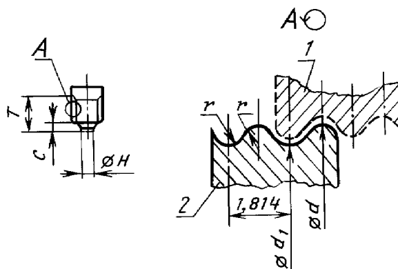
1 — патрон; 2 — цоколь
