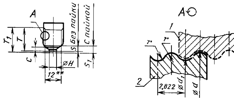
1 — патрон; 2 — цоколь
