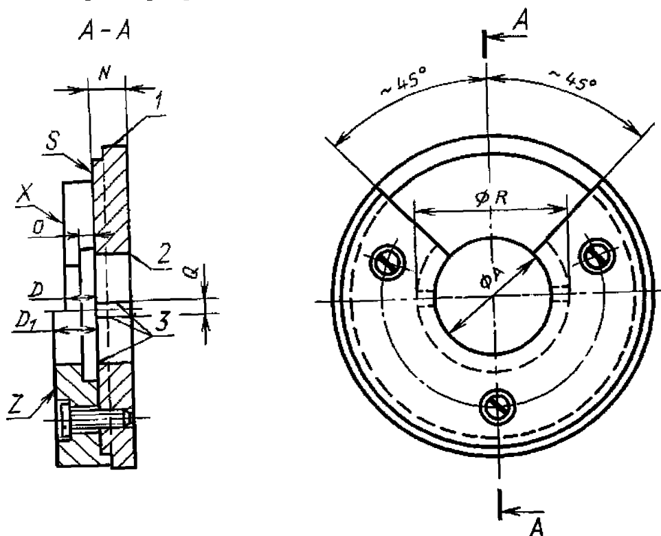
1 — накатка; 2 — кромка острая; 3 — кромки слегка скошены
