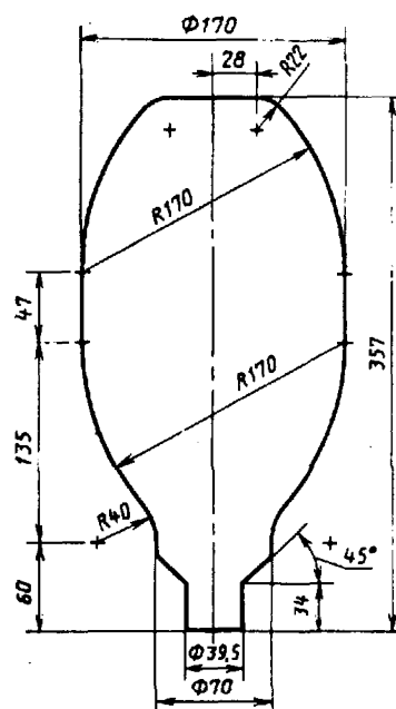
Наибольший контур ртутной лампы высокого давления мощностью 700 Вт с цоколем E40
