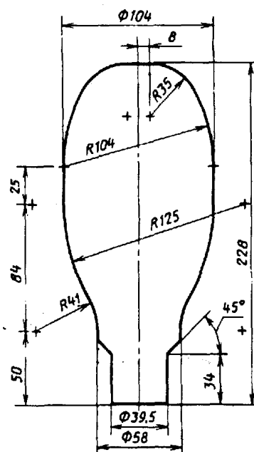
Наибольший контур ртутной лампы высокого давления мощностью 175 и 250 Вт
