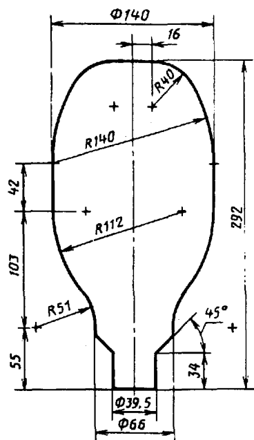
Наибольший контур ртутной лампы высокого давления мощностью 400 Вт
