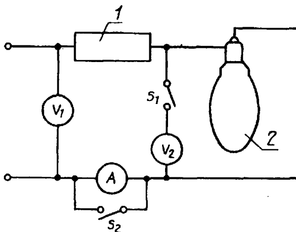
1 — балласт; 2 — лампа
