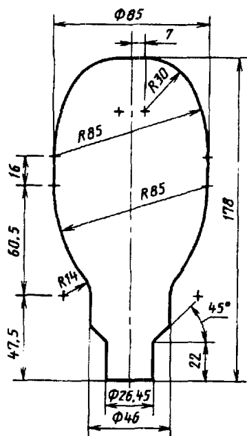
Наибольший контур ртутной лампы высокого давления мощностью 125 Вт
