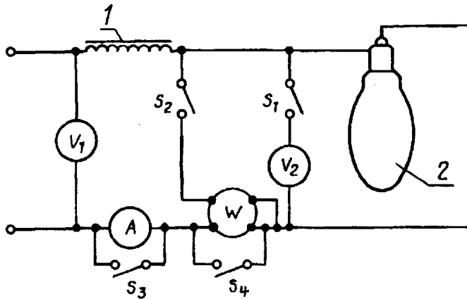
1 — образцовый балласт; 2 — лампа
