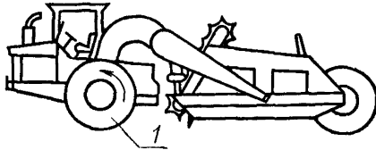
1 — ведущие колеса Черт. 9
