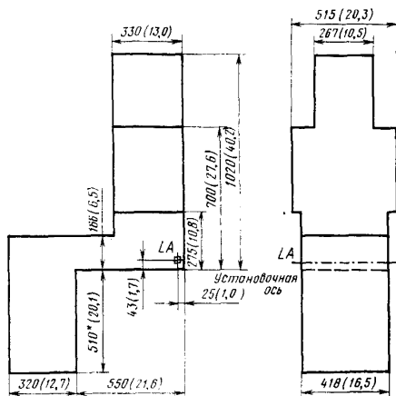
Объем ограничения деформации (DLV) Размеры в мм
