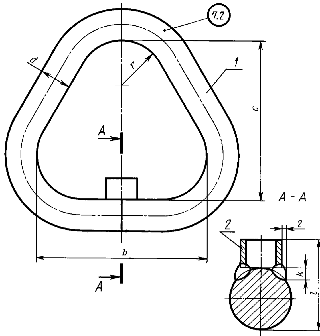
1 — подвеска; 2 — упор
