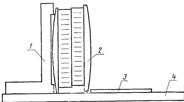
1—угловая плита; 2—блок; 3—щуп; 4—поверочная плита
