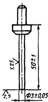
Рисунок 1 — Пестик к прибору Вика
