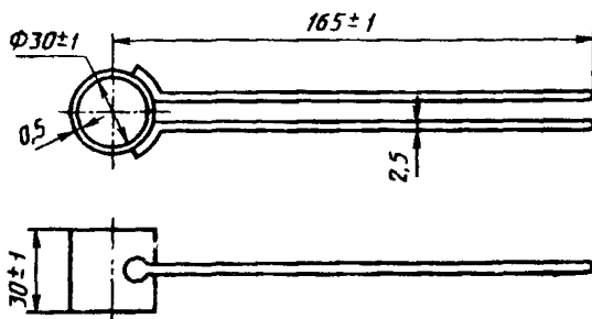
Рисунок 2 — Кольцо Ле-Шателье
