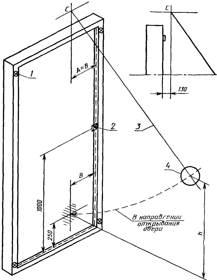
1 — прижим; 2 — запирающий прибор или ограничитель; 3 — гибкая нить; 4 — неупругое тело (груз). B = 1/3 ширины полотна, но не более 300 мм.
