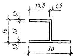
Профиль ПС 885—266
