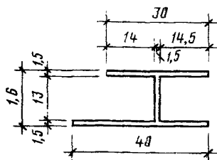
Профиль ПС 885—267
