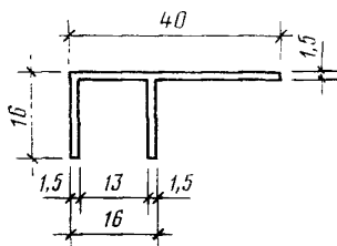
Профиль ПС 885—265
