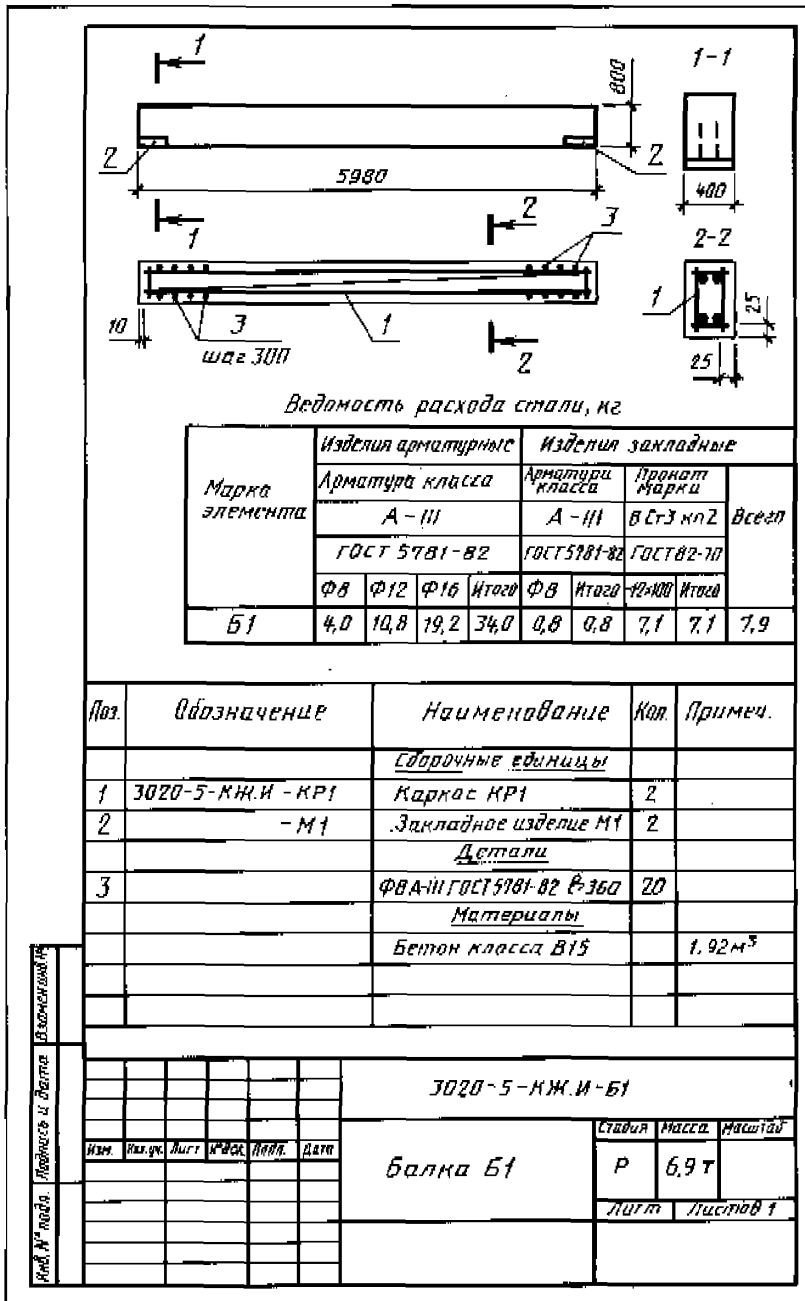
Пример выполнения чертежа индивидуального изделия
